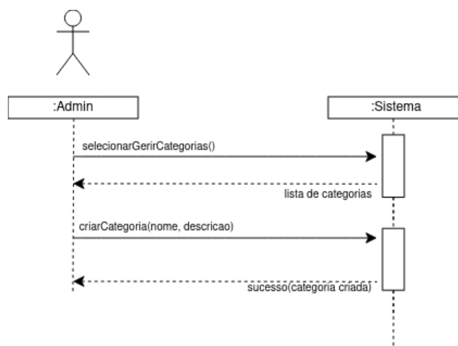
Fig. 10. UC07: Gerir CATEGORIAS
