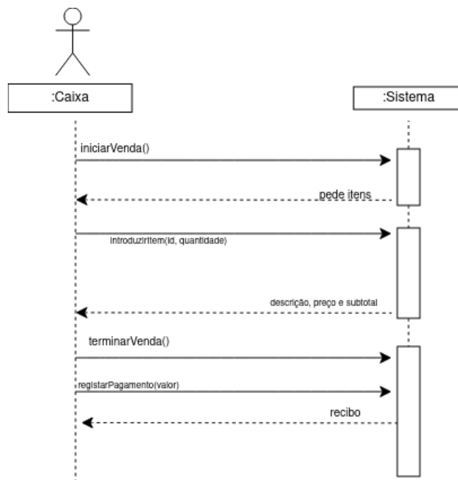
Fig. 11. UC08: Realizar VENDA
