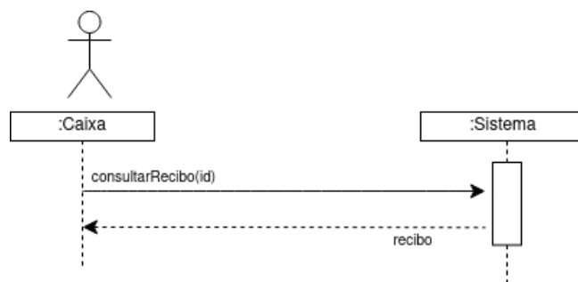
Fig. 16. UC13: Consultar RECIBO
