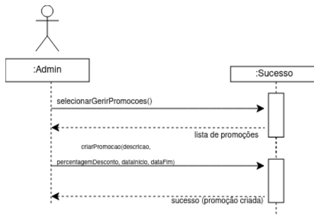
Fig. 9. UC06: Gerir PROMOÇÕES (Cenário de Criação)
