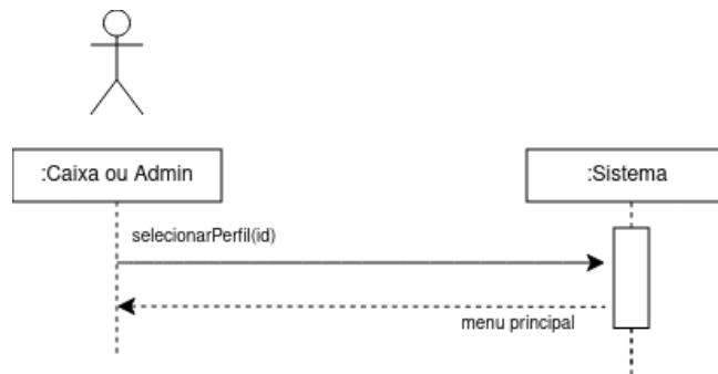
Fig. 17. UC14: Selecionar Perfil
