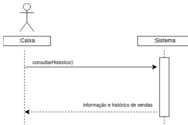
Fig. 13. UC10: Ver Info Própria
