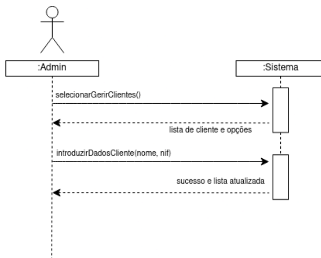
Fig. 8. UC05: Gerir CLIENTES (Cenário de Registo)
