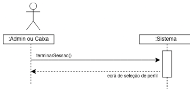
Fig. 18. UC15: Sair do Perfil
