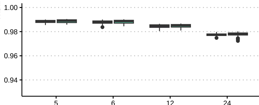
Cues: Politics
