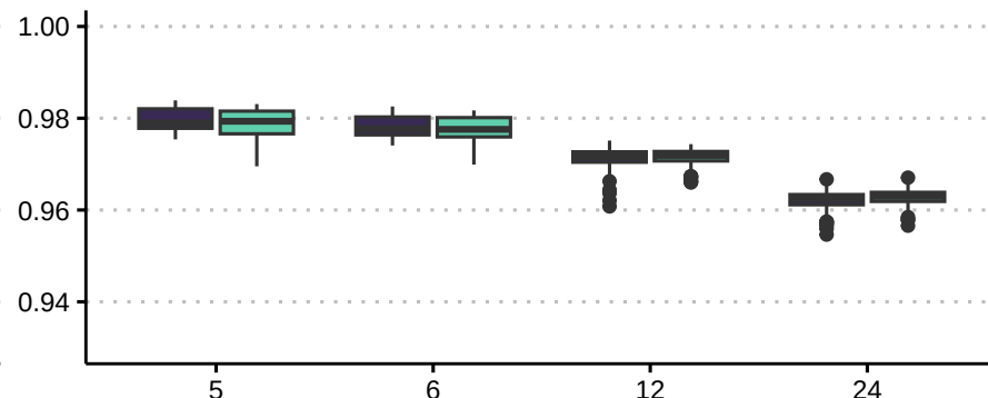
Cues: Sports
