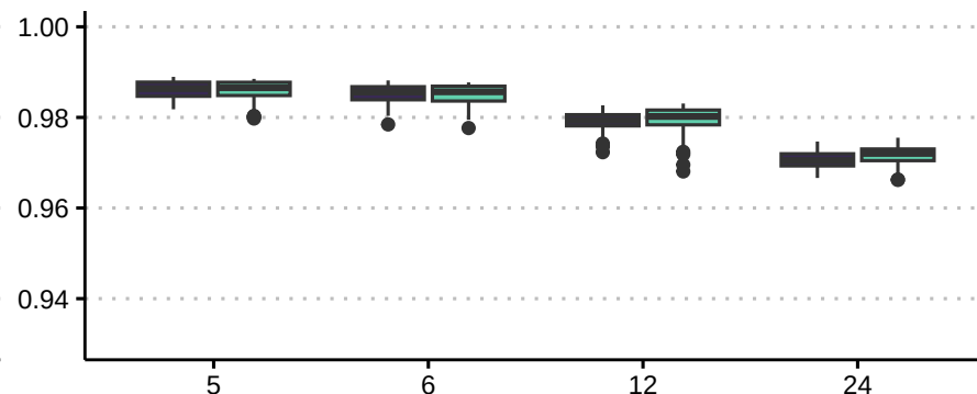
Cues: Random
