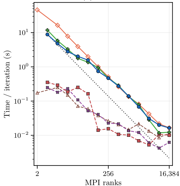
(a) Poisson
