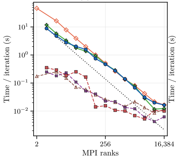
(a) Poisson
