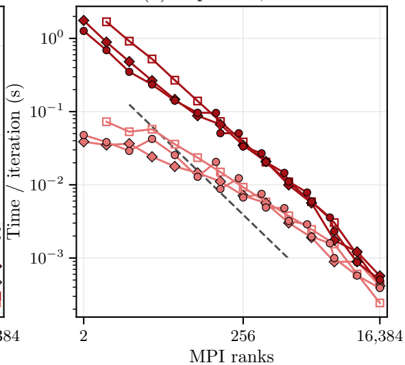
(d) Laplacian, L = 9
