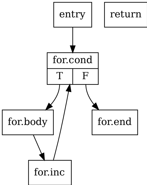
CFG for 'bar' function
