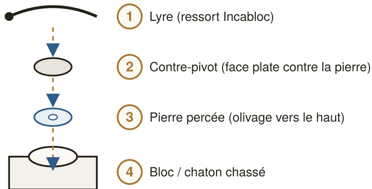
Antichoc — ordre de dépose et orientation des pierres
