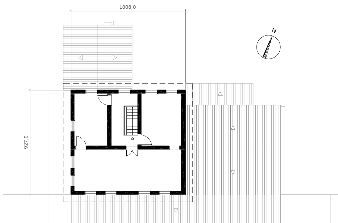
Planta do segundo pavimento.
