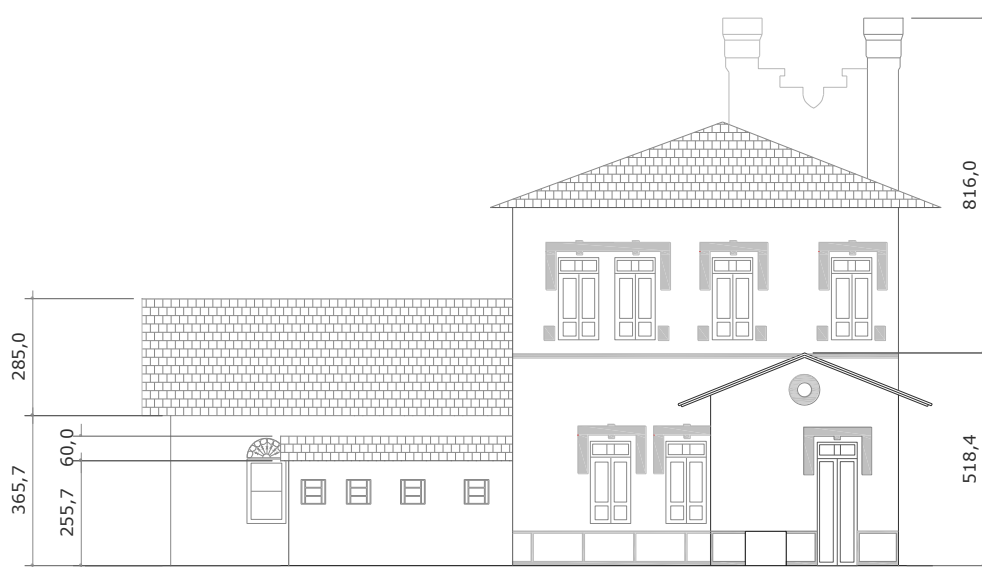
Fachada posterior.
