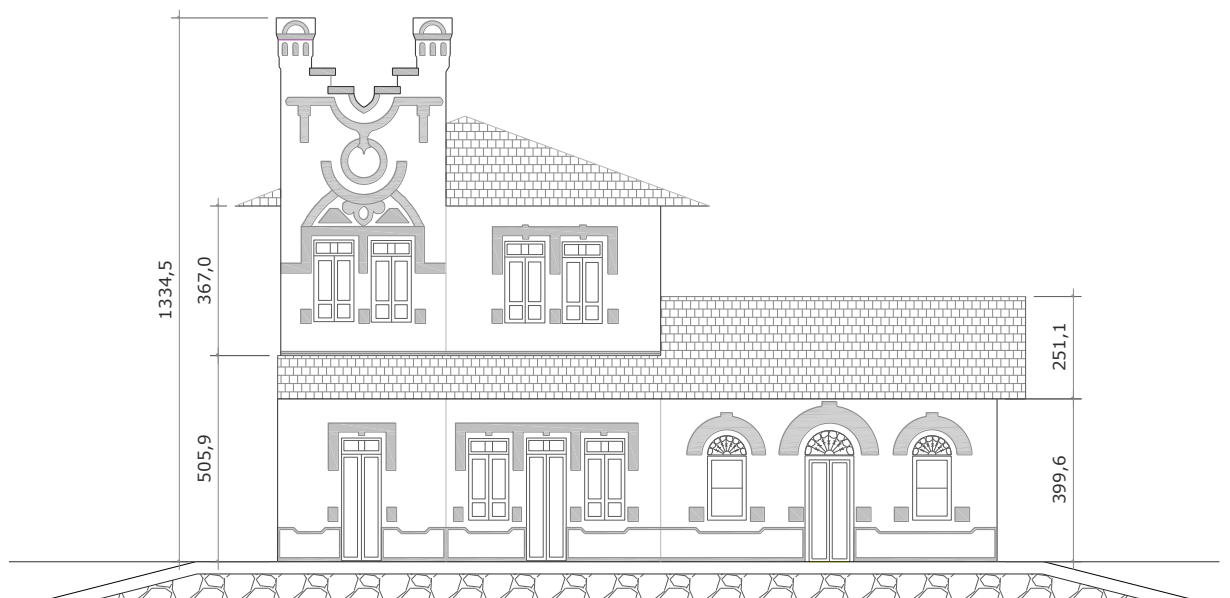
Fachada frontal.
