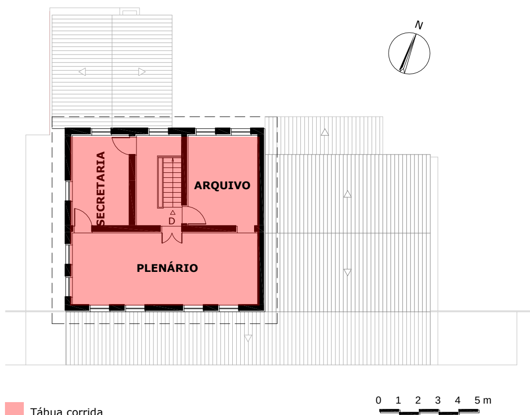
Planta de piso do segundo pavimento. Desenho: Sofia Cunha, mar/2008.
