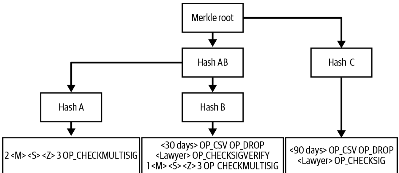
Figure 41. MAST yenye hati ndogo tatu.
