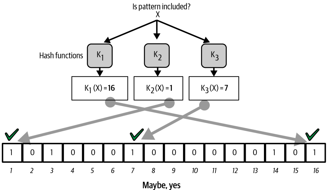
Figure 55. Kujua uwepo wa mfumo "X" katika kichujio cha bloom. Matokeo ni mechi chanya ya uwezekano, inayomaanisha "Labda."
