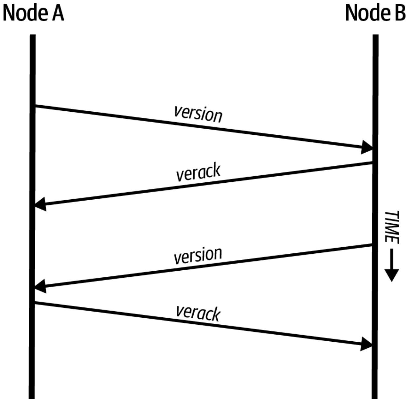
Figure 49. Msalimiano wa awali kati ya rika.
