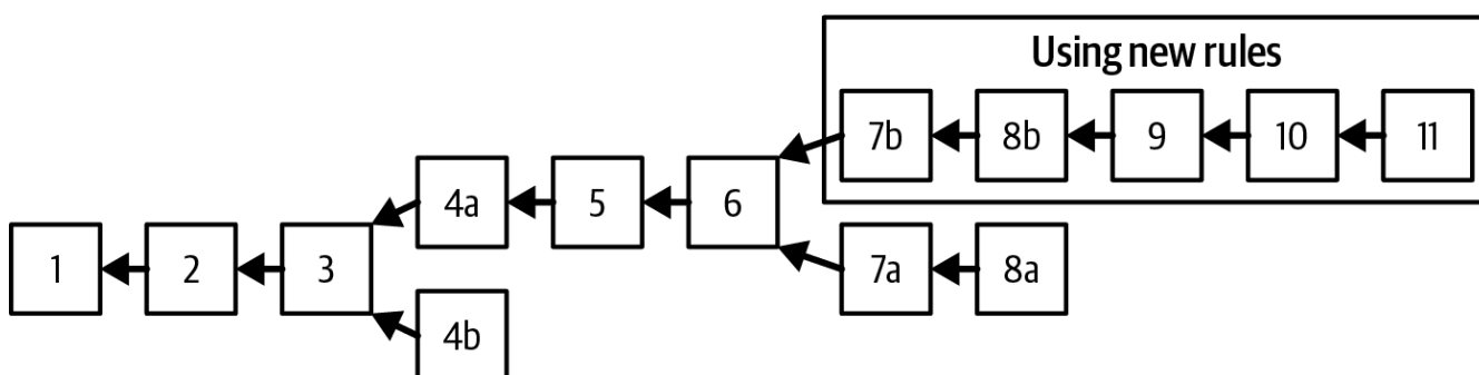
Figure 64. Mnyororo wa vitalu wenye matawi.
