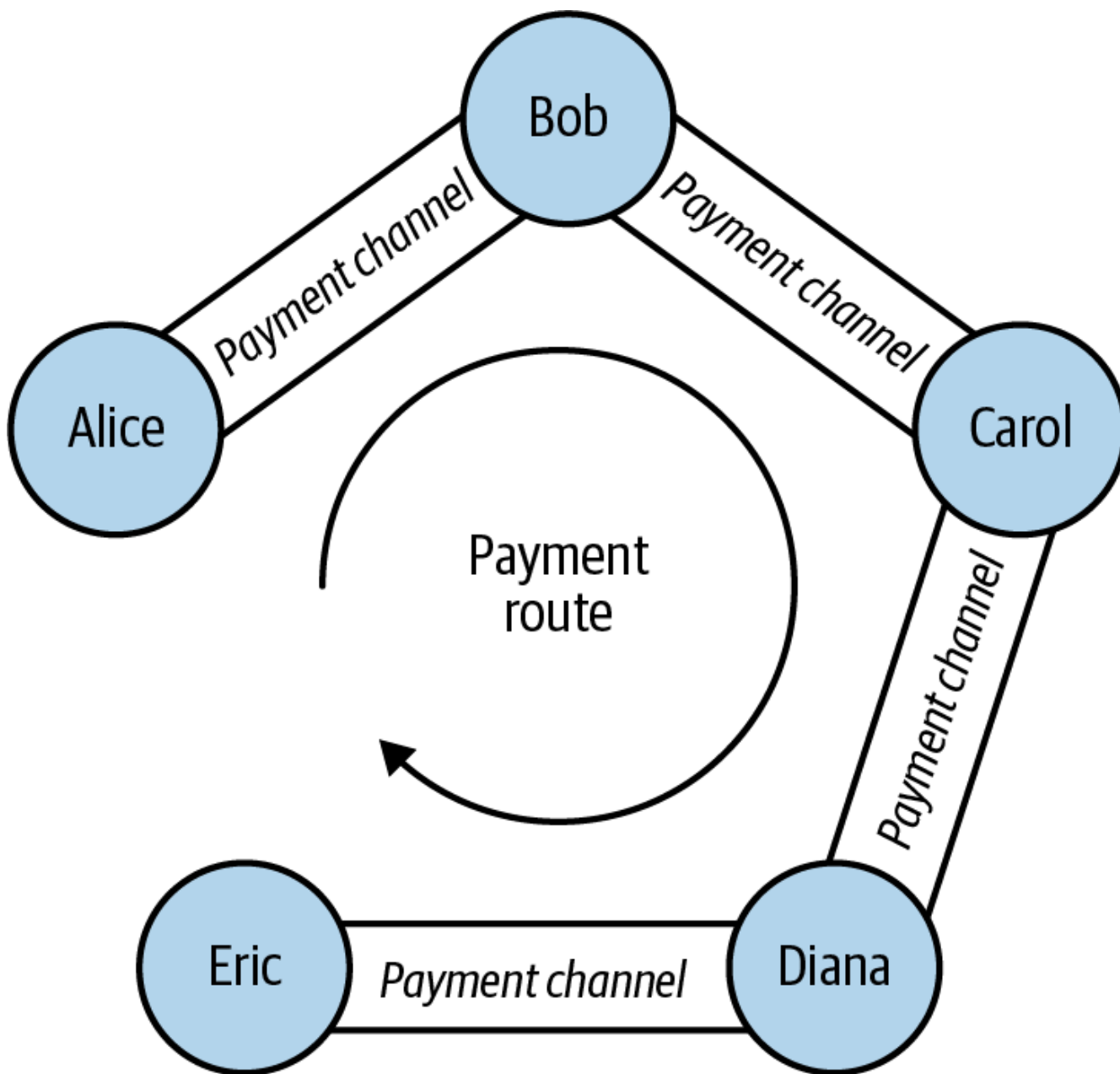
Figure 71. Mfululizo wa njia za malipo za pande mbili zilizounganishwa kuunda LN ambayo inaweza kuelekeza malipo kutoka Alice hadi Eric.
