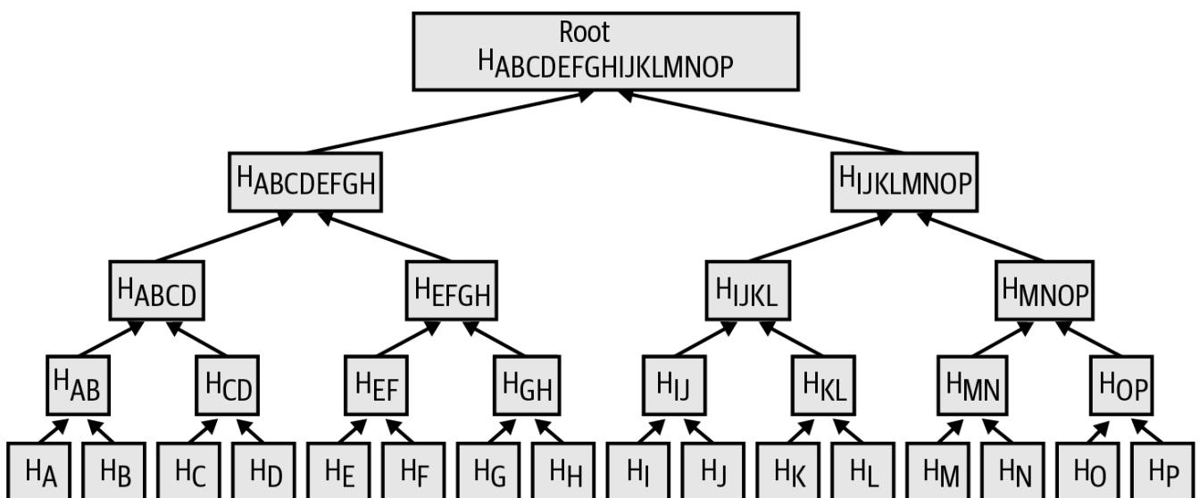
Figure 61. Mti wa merkle ukimuhtasiri vipengele vingi vya data.
