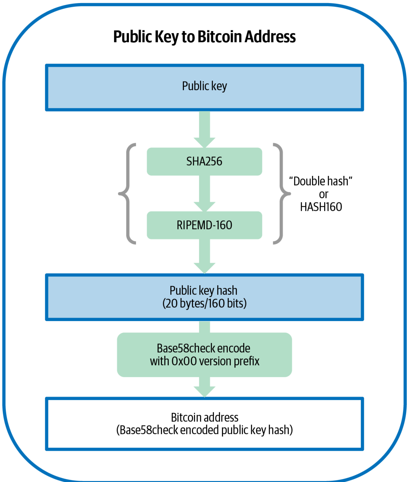
Figure 18. Funguo ya umma hadi anwani ya Bitcoin: ubadilishaji wa funguo ya umma kuwa anwani ya Bitcoin.
