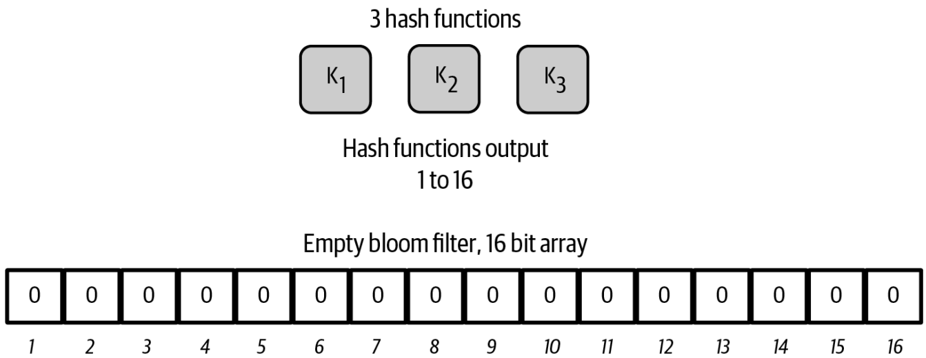
Figure 52. Mfano wa kichujio rahisi cha bloom, chenye sehemu ya biti 16 na vitendakazi vitatu vya hash.
