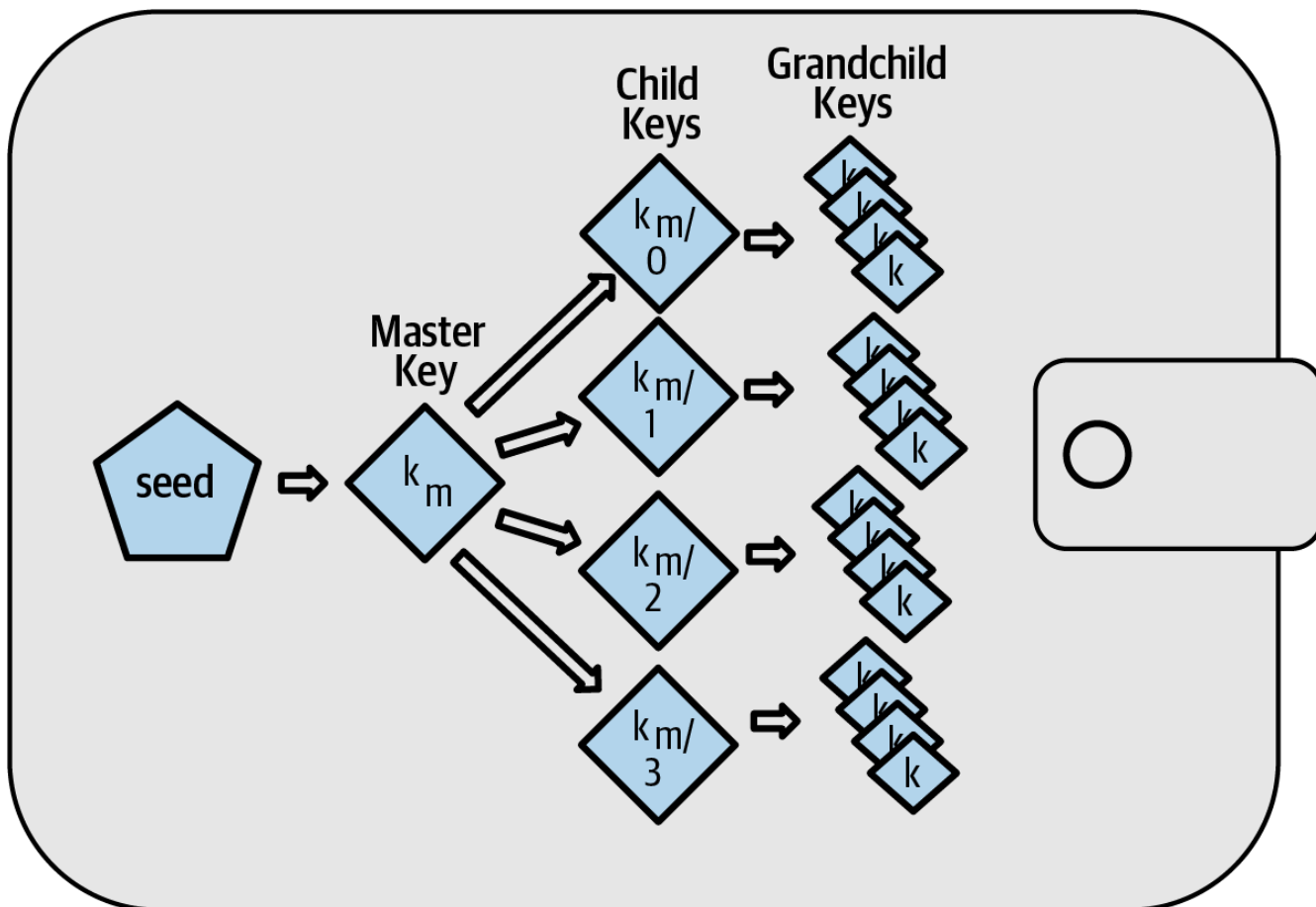
Figure 24. Mkoba wa HD: mti wa funguo uliozalishwa kutoka mbegu moja.
