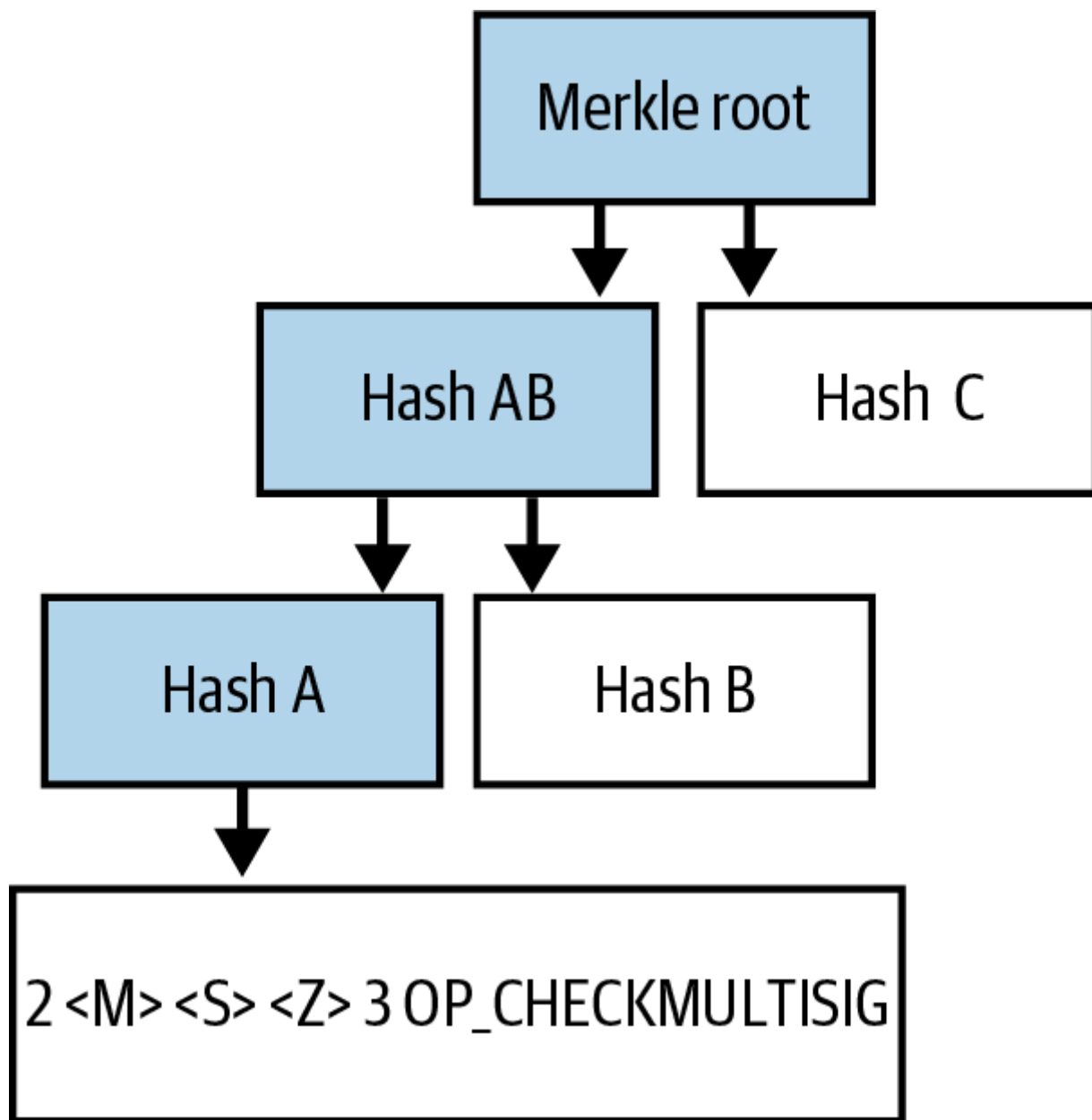
Figure 42. Uthibitisho wa ushirika wa MAST kwa moja ya hati ndogo.
