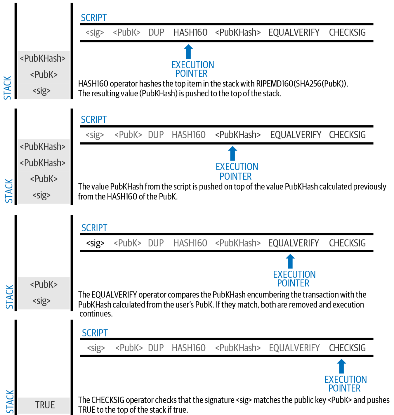
Figure 40. Kutathmini hati kwa muamala wa P2PKH (sehemu 2 ya 2).
