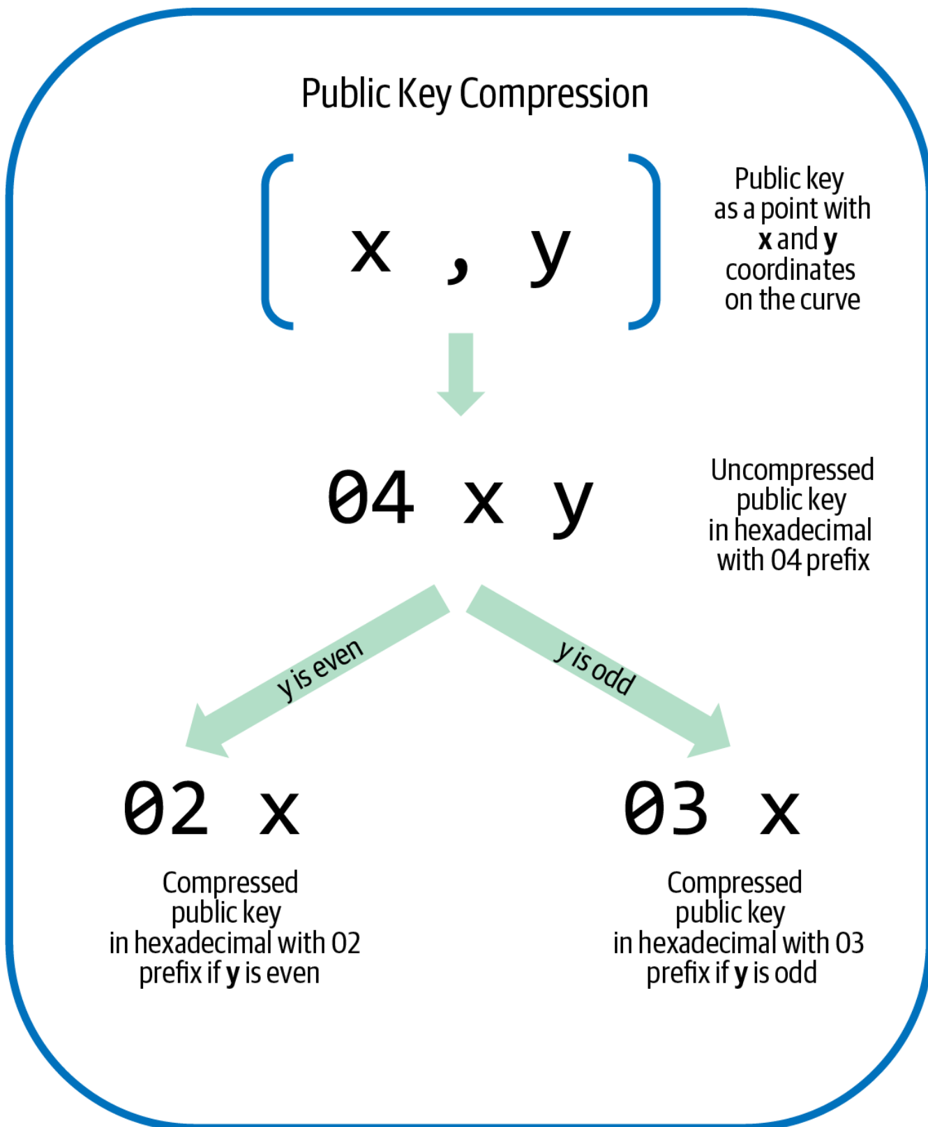
Figure 19. Usongaji wa funguo ya umma.
