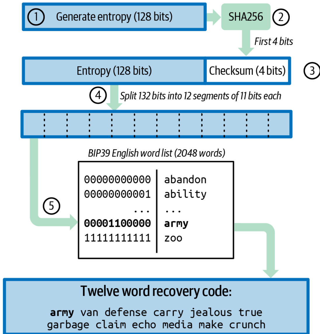
Figure 25. Kuzalisha entropi na kuisimba kama msimbo wa urejeshaji.
