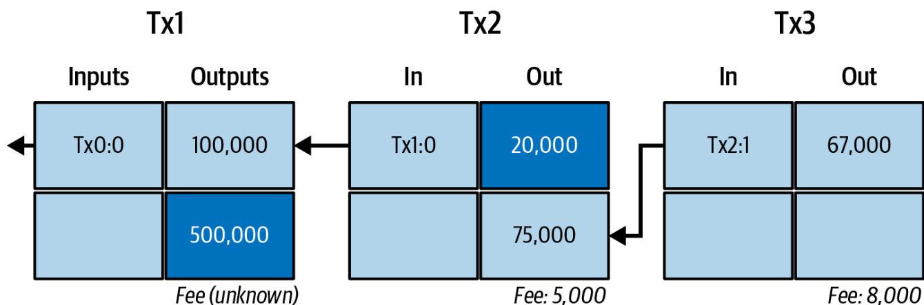
Figure 5. Mnyororo wa miamala, ambapo matokeo ya muamala mmoja ndiyo ingizo la muamala unaofuata.
