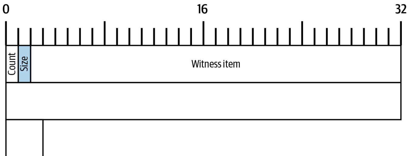
Figure 35. Ramani ya baiti ya muundo wa shahidi wa muamala wa Alice.
