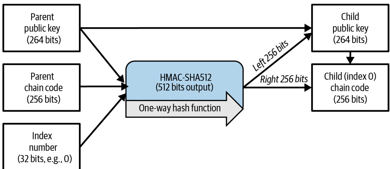
Figure 29. Kupanua funguo ya umma ya mzazi kuunda funguo ya umma ya mtoto.
