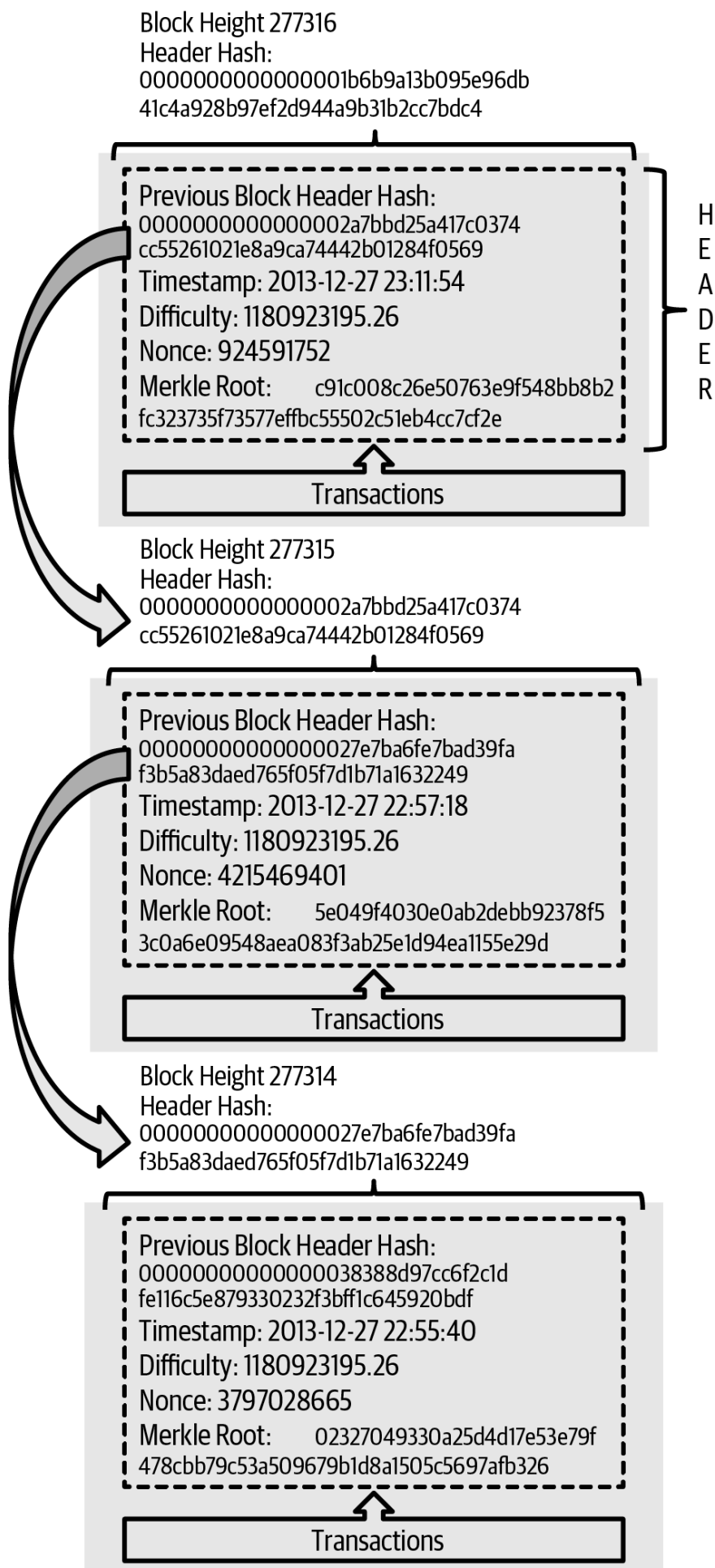
Figure 57. Vitalu vilivyounganishwa katika mnyororo, kila kimoja kikirejelea hash ya kichwa cha kitalu kilichotangulia.
