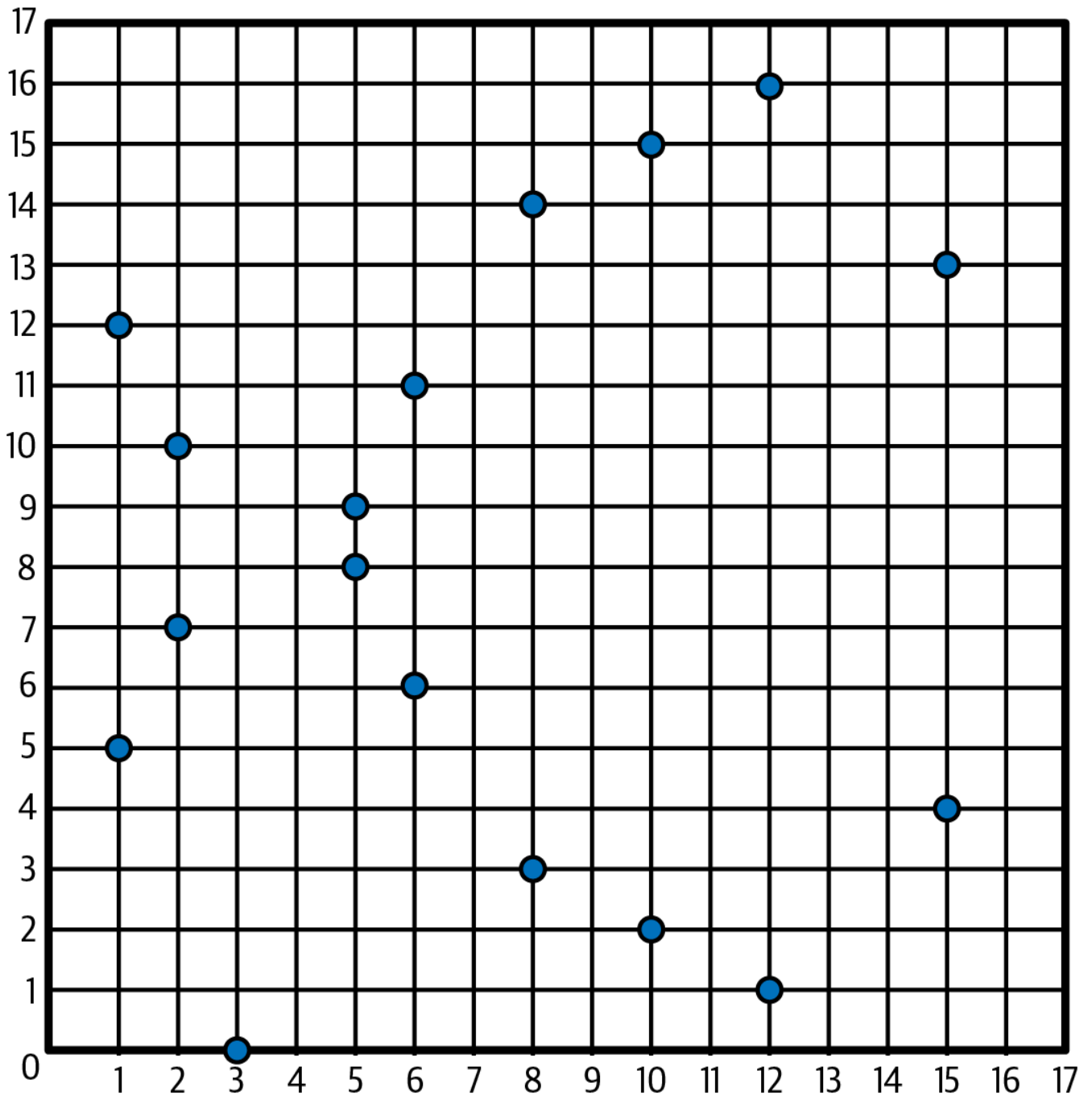
Figure 14. Kriptografia ya mzunguko wa mviringo: kuibua mzunguko wa mviringo juu ya F(p) , ambapo p=17 .
