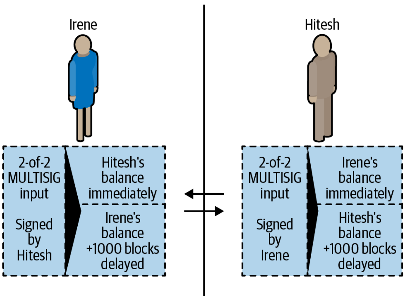
Figure 70. Miamala miwili ya ahadi ya asymmetric yenye malipo yaliyocheleweshwa kwa chama kinachoshikilia muamala.
