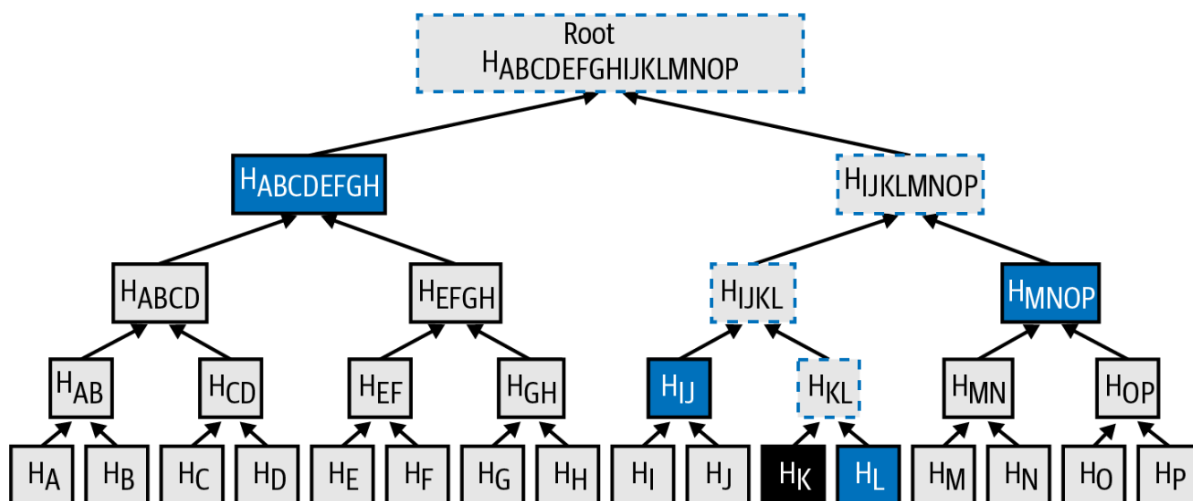
Figure 62. Njia ya merkle inayotumiwa kuthibitisha kujumuishwa kwa kipengele cha data.
