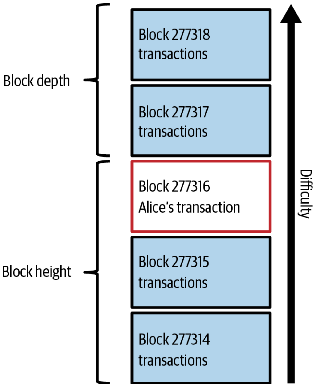
Figure 9. Muamala wa Alice umejumuishwa katika kizuizi.
