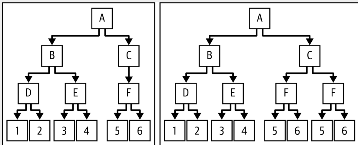
Figure 60. Miti miwili ya merkle ya mtindo wa Bitcoin yenye mzizi sawa lakini idadi tofauti ya majani.
