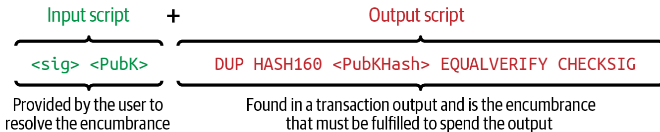
Figure 37. Kuunganisha hati za pembejeo na tokeo kutathmini hati ya muamala.
