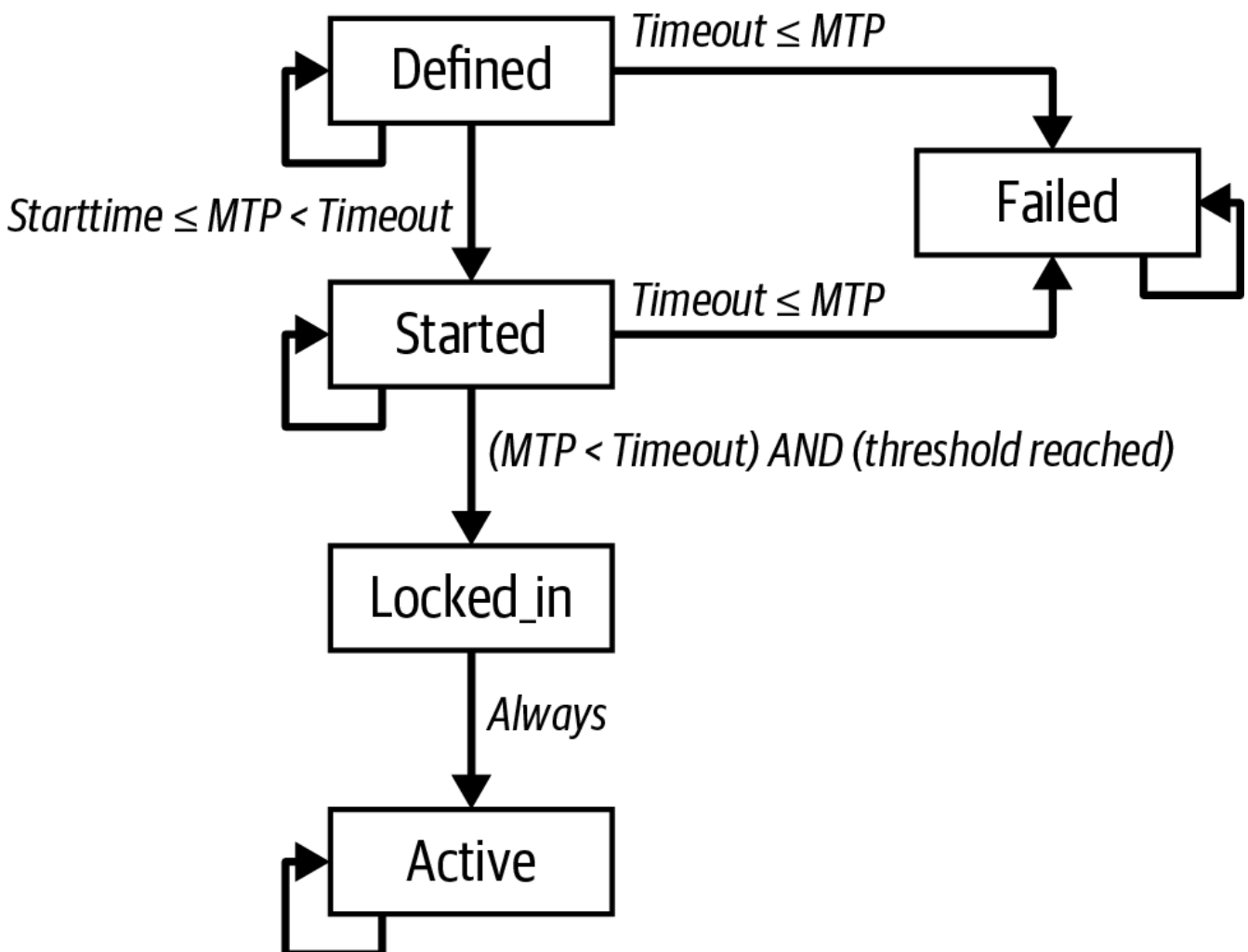
Figure 65. Mchoro wa mabadiliko ya hali ya BIP9.
