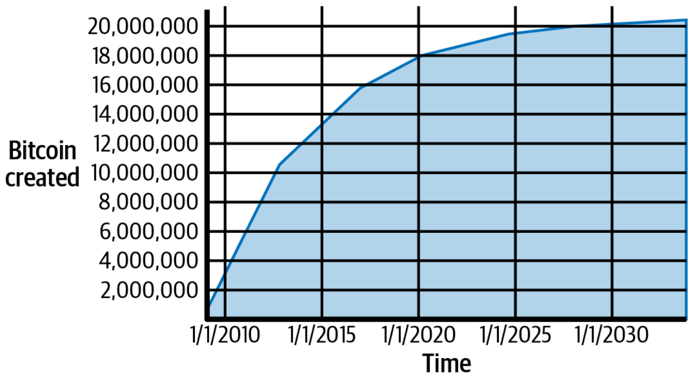
Figure 63. Ugavi wa sarafu ya bitcoin kwa wakati kulingana na kiwango cha utoaji kinachopungua kijiometri.
