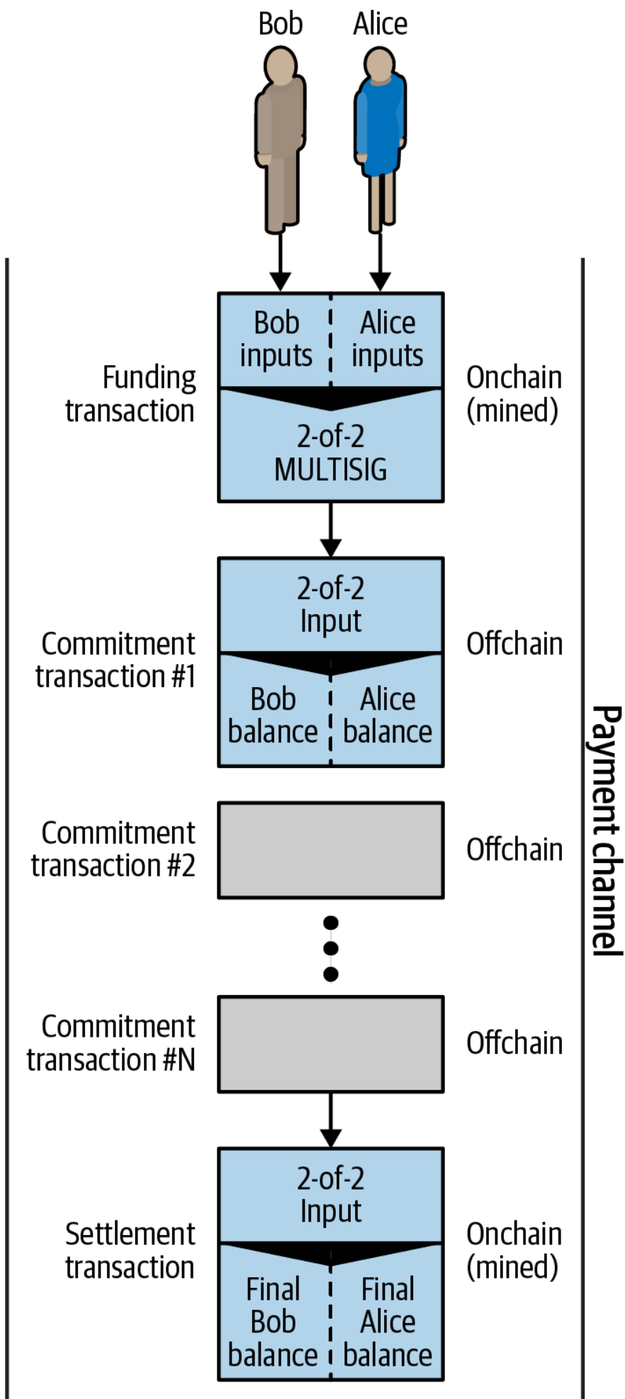
Figure 66. Njia ya malipo kati ya Bob na Alice, ikionyesha miamala ya ufadhili, ahadi, na usuluhishi.
