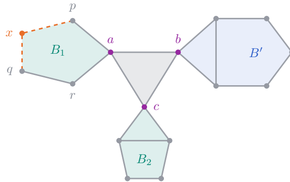
граф связности 1 с \delta \geq 2 : крайние блоки B_1, B_2 размера m = 5 (так что k = 2 ) и B' размера 6; точки сочленения a, b, c . После удаления x \in \text{Int}(B_1) от блока B_1 остаётся путь parq , и r — новая точка сочленения
