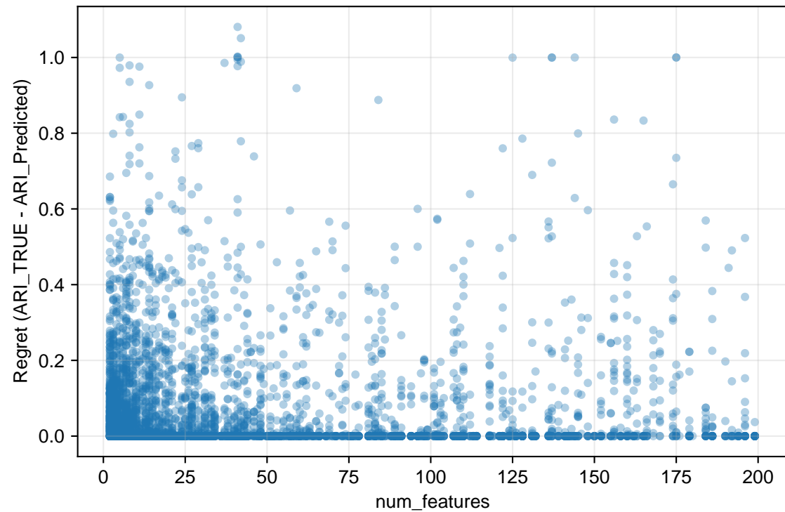
Regret vs #Features (d) Spearman \rho = -0.128
