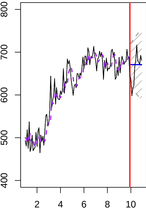
ETS(A,N,N)
