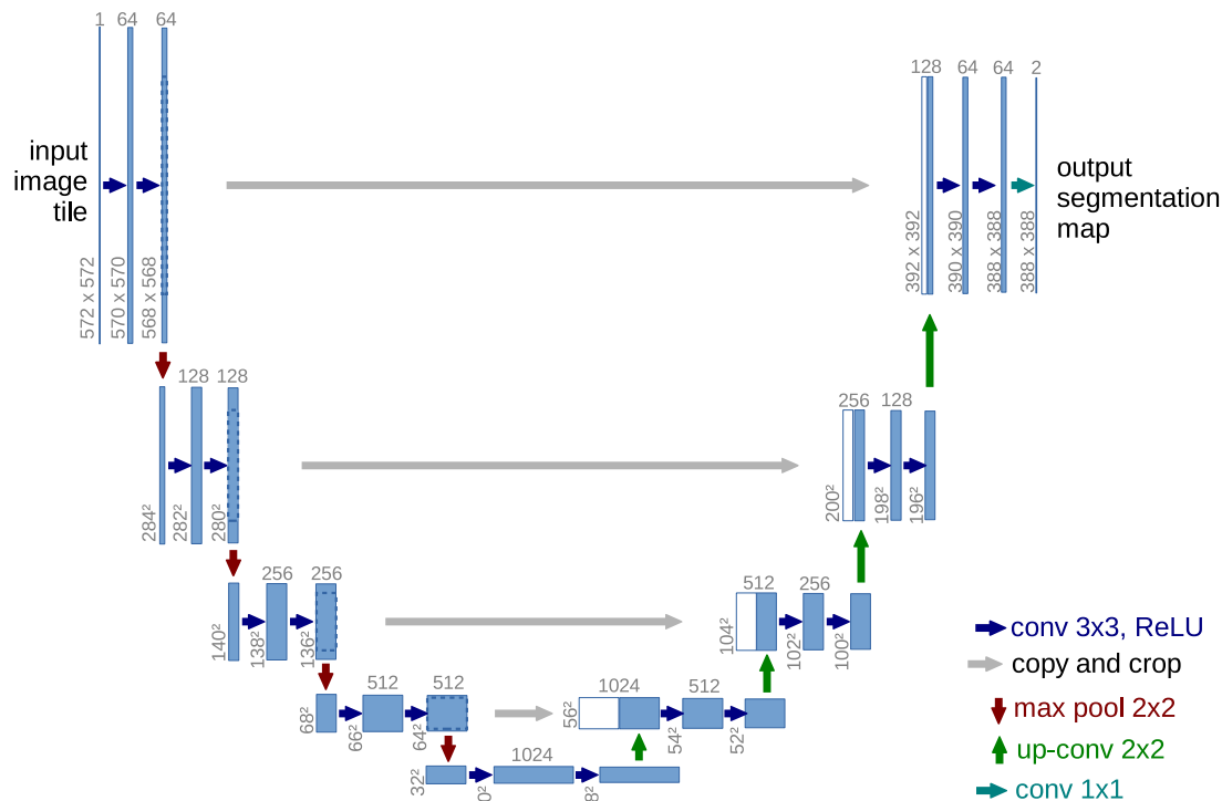
图 4.18 U-net 模型
