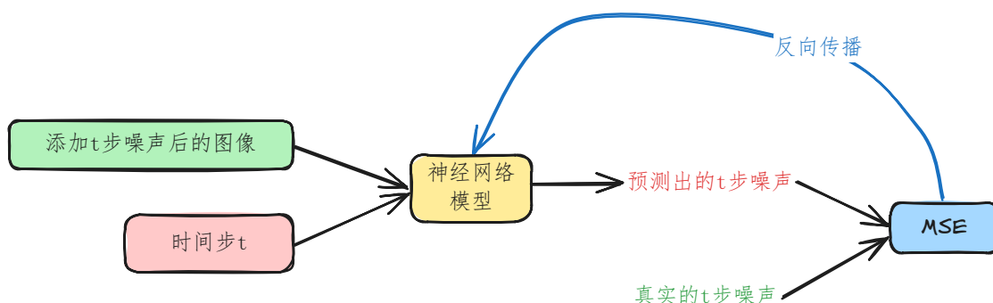
图 3.16 以噪声为预测目标
