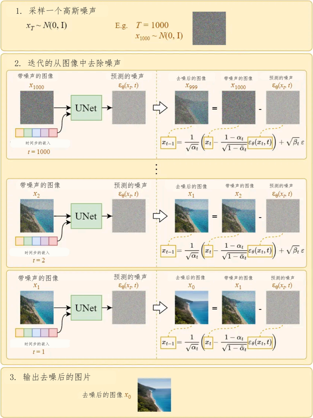
图 3.15 扩散模型的采样过程
