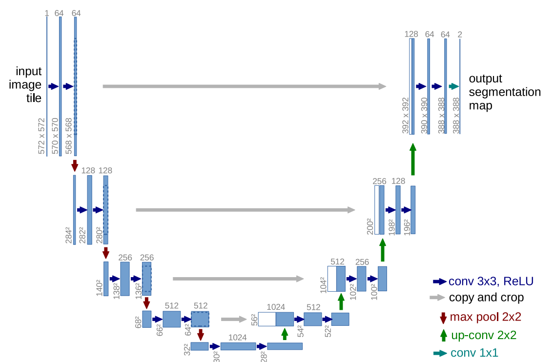
图 3.6 U-net 架构（以最低分辨率为 32\times32 像素为例）。每个蓝色方框对应一个多通道特征图。方框顶部标注了通道数量。方框左下角标注了 x - y 尺寸。白色方框表示复制的特征图。箭头表示不同的操作。
