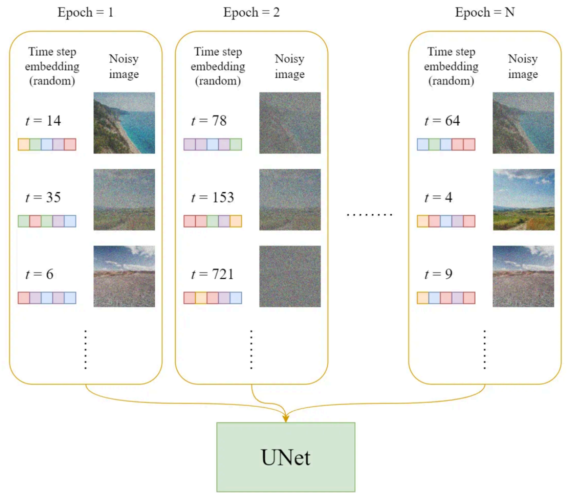
图 3.11 训练 unet
