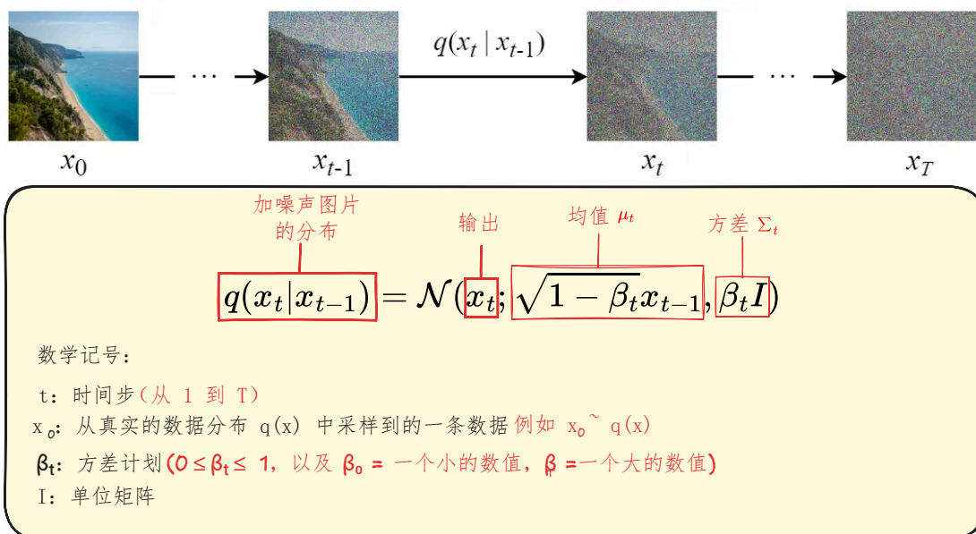
图 3.9 正向扩散公式图解
