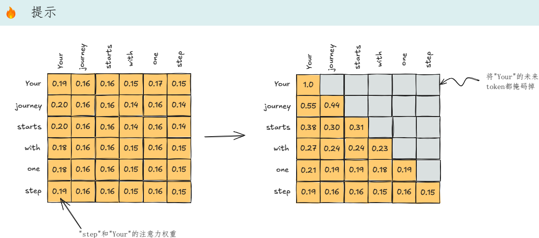
图 2.6 因果注意力分数的掩码
