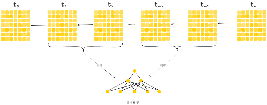
图 3.7 共享模型
