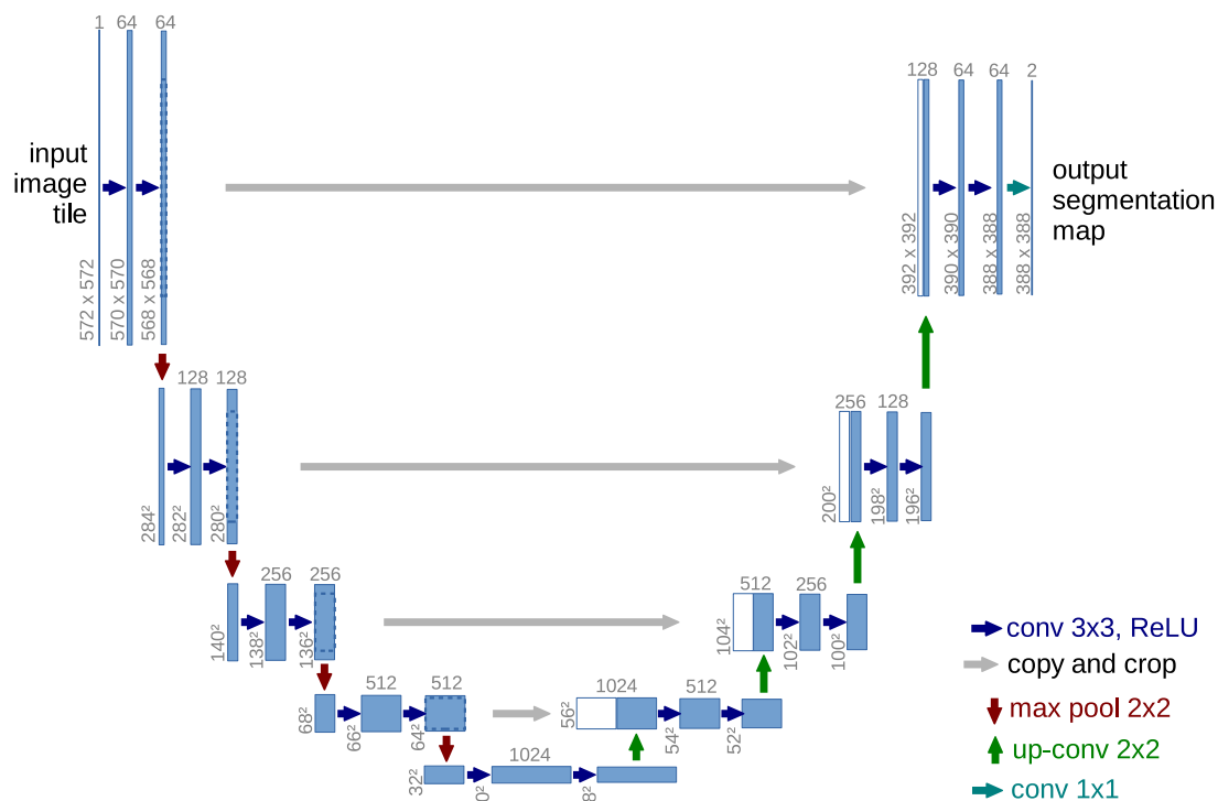
图 3.18 U-net 模型
