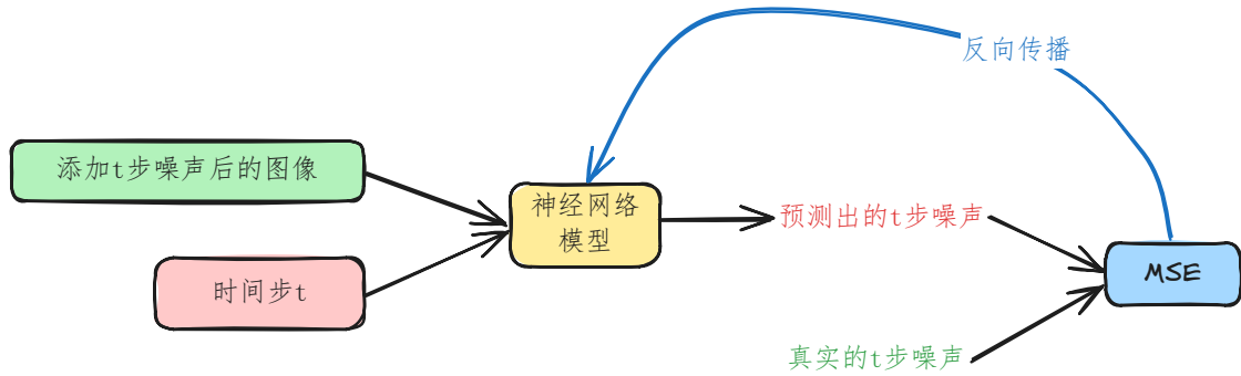
图 3.10 以噪声为预测目标
