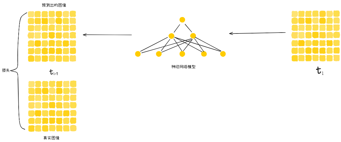
图 4.4 预测图像与实际图像之间的差异使用损失函数计算
