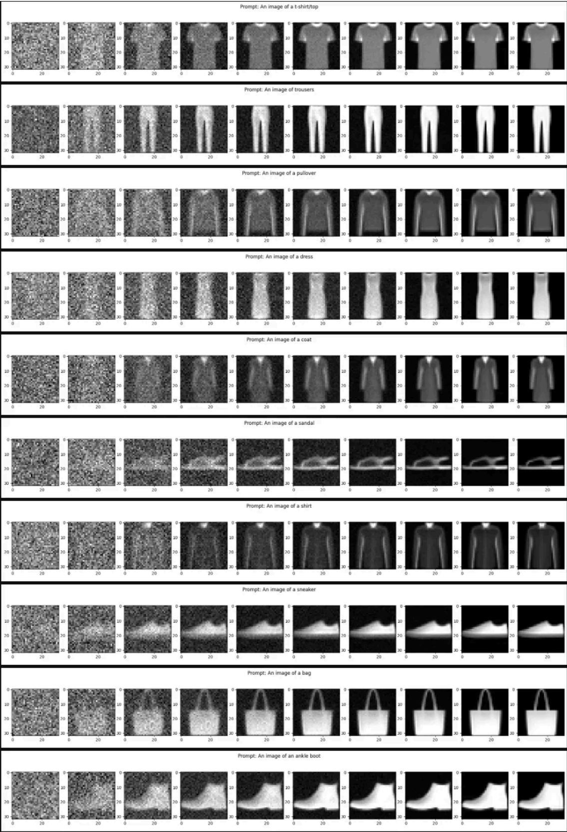
图 7.8 训练结果
