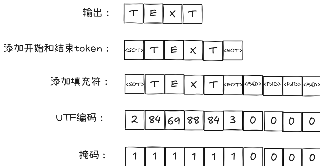
图 2.3 分词过程
