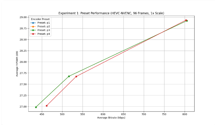
图 4.7 NVENC 编码预设对比实验 (HEVC-NVENC, 96 帧, 1x Scale)
