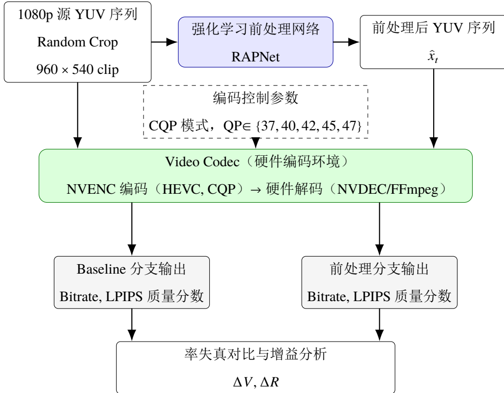
图 3.1 总体前处理流程图
