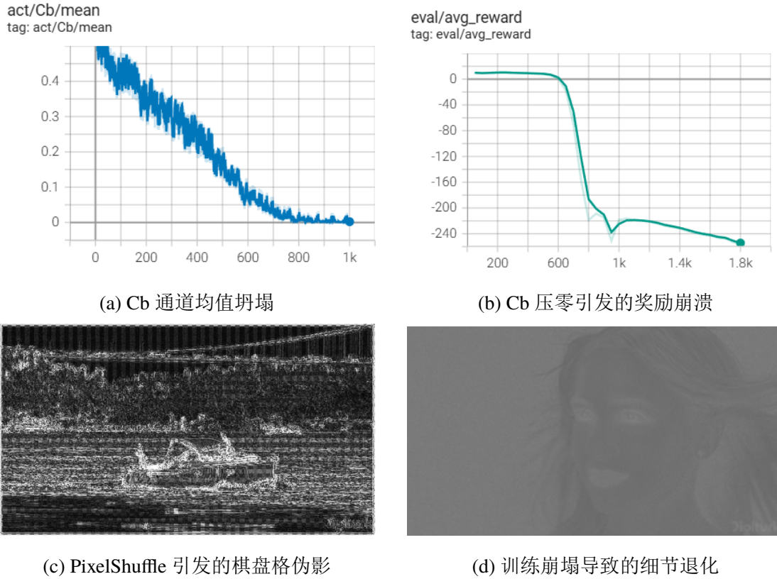
图 4.3 训练过程中的典型失败案例
