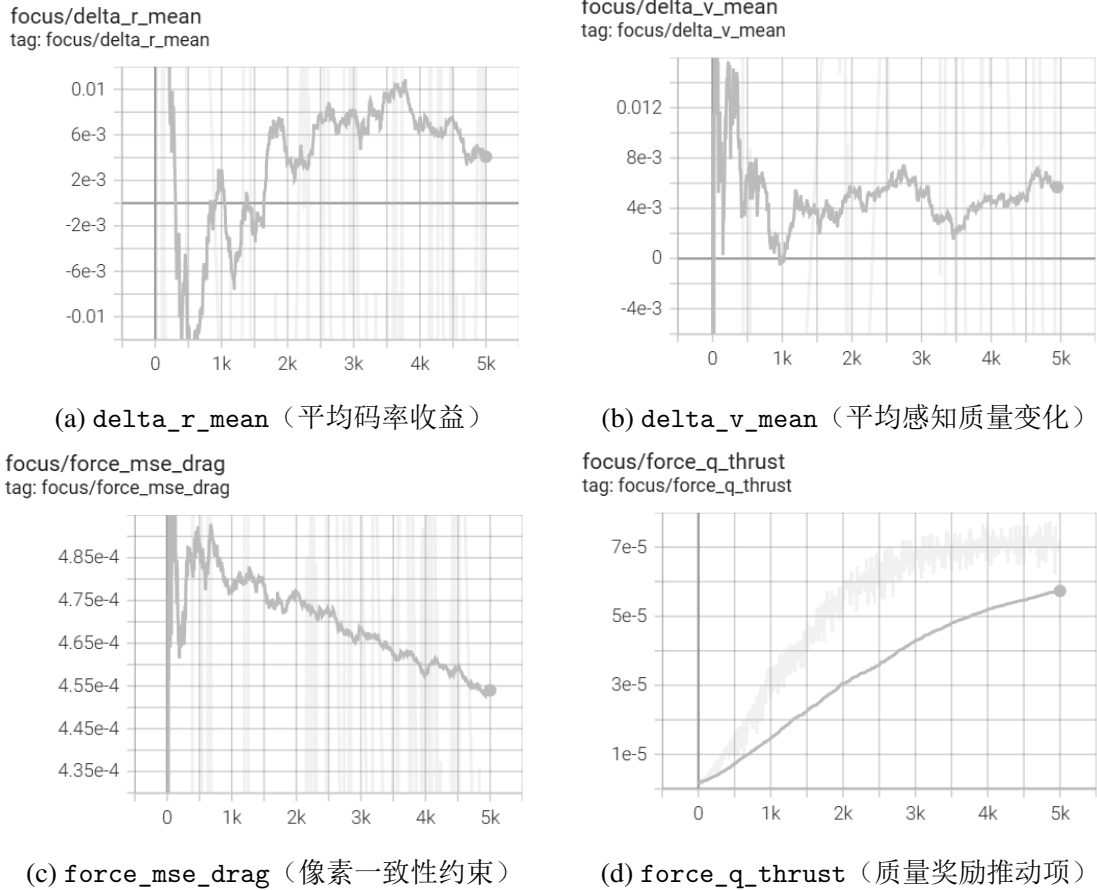
图 4.2 TensorBoard 训练监控关键曲线
