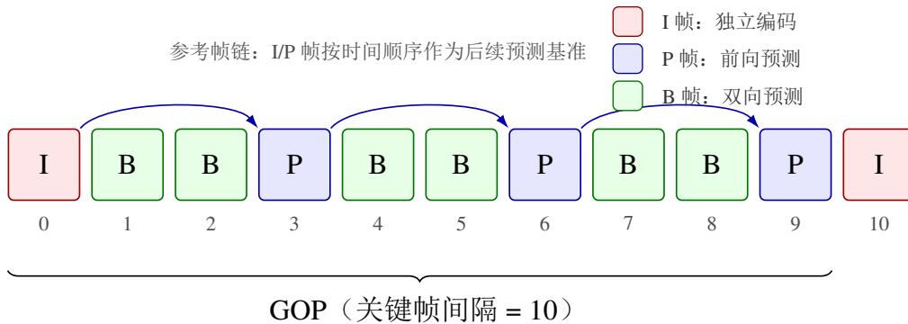
图 2.1 I/P/B 帧类型与 GOP 结构示意图
