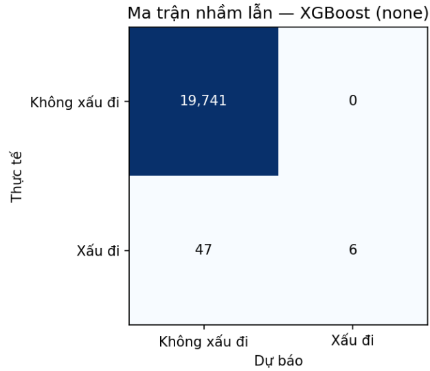
Hình 3.1: Ma trận nhầm lẫn — XGBoost (none), tập kiểm định minh họa
