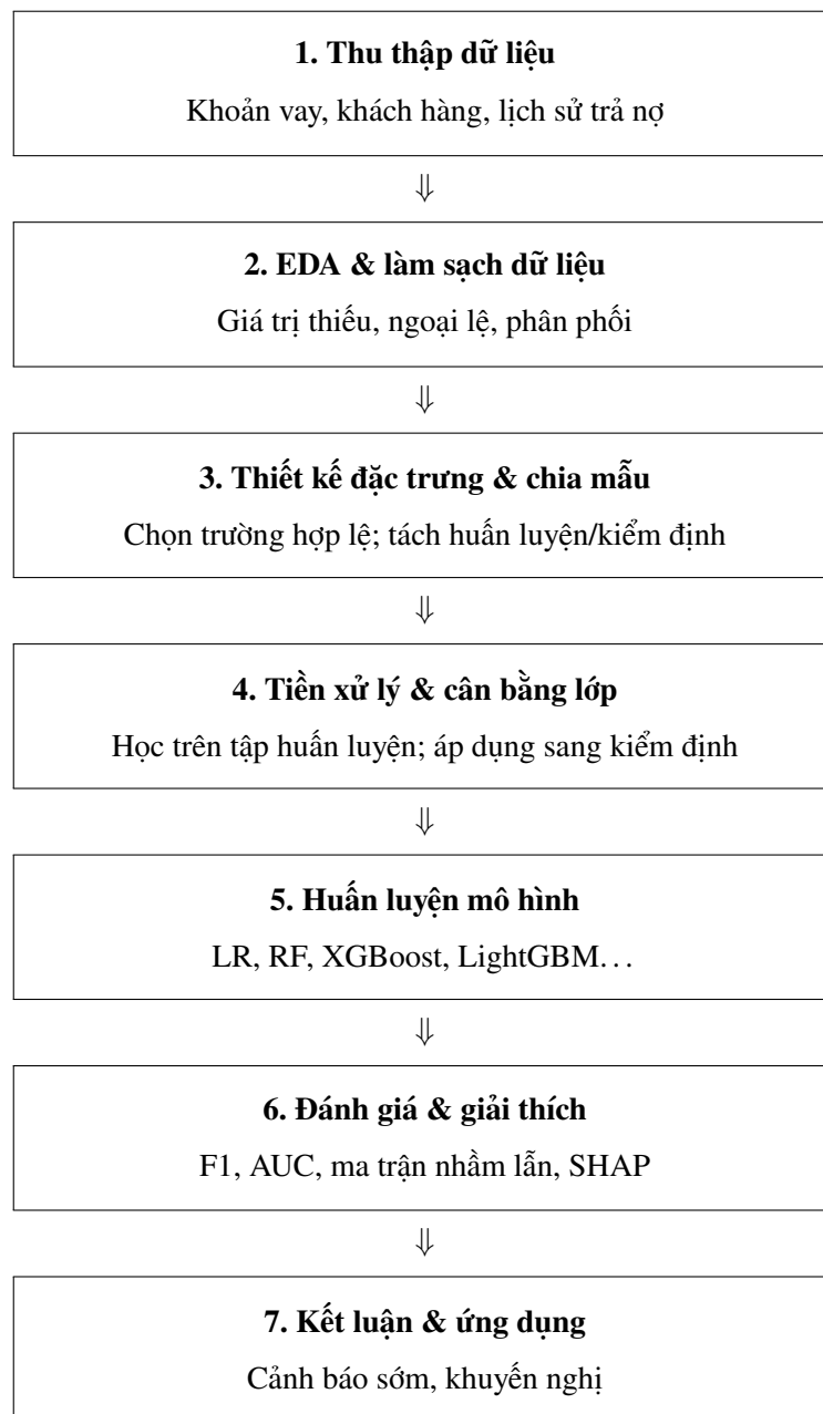
Hình 2.1: Pipeline nghiên cứu tổng thể — từ thu thập dữ liệu tới kết luận và ứng dụng
