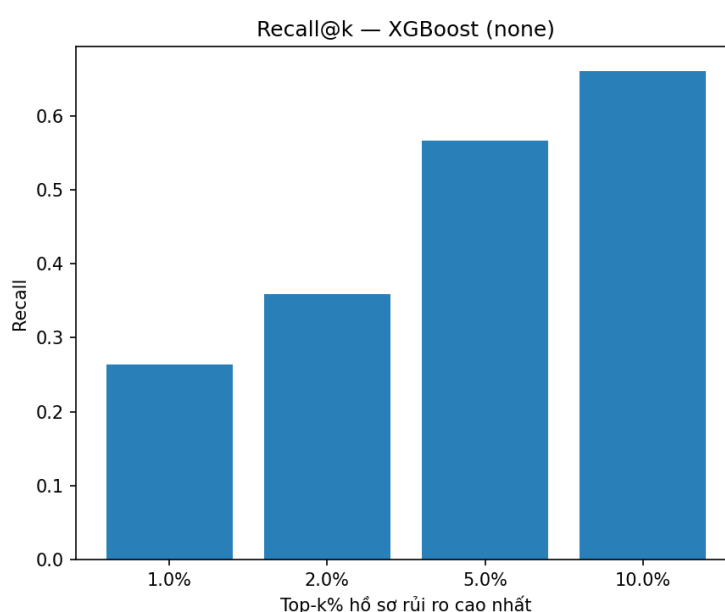
Hình 3.3: Recall@k — XGBoost (none)
