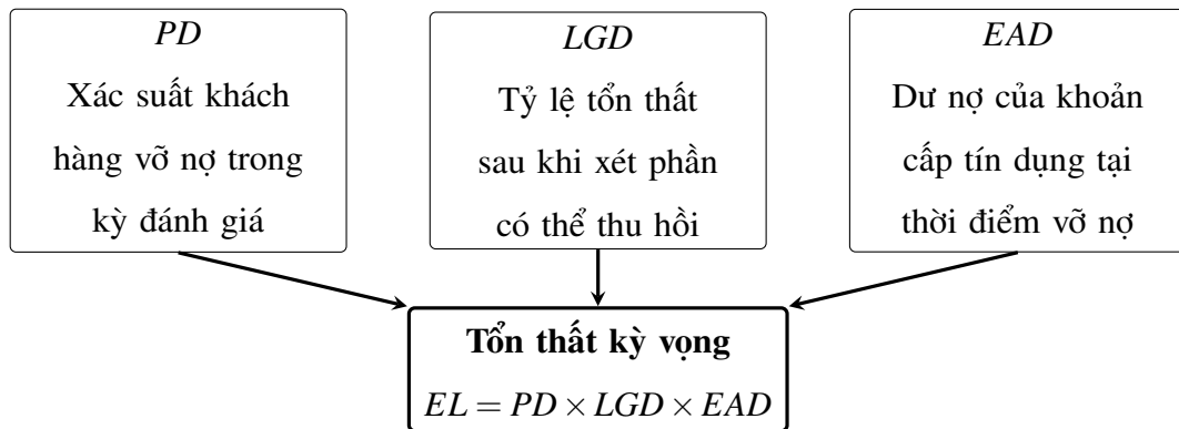
Hình 1.1: Các cấu phần của tổn thất kỳ vọng trong rủi ro tín dụng
