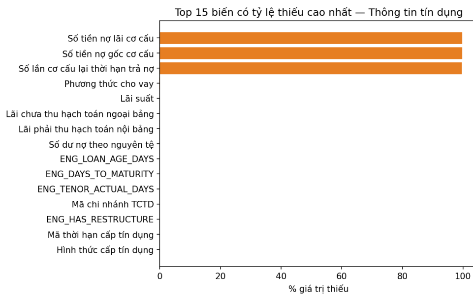
Hình 2.5: Top 15 biến (trong bể đặc trưng hợp lệ) có tỷ lệ thiếu cao nhất — bộ dữ liệu B
