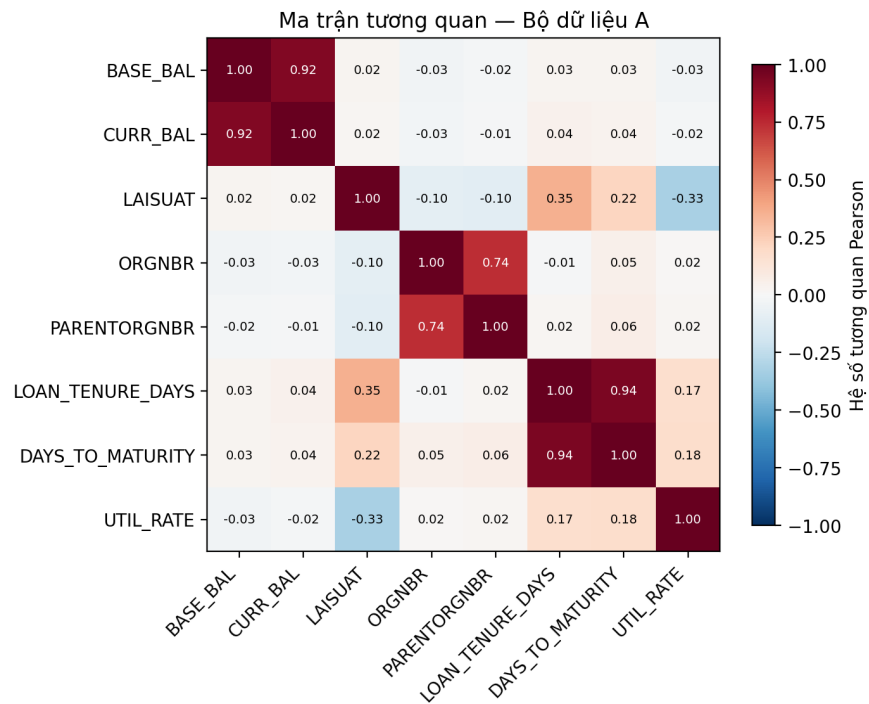
Hình 2.3: Ma trận tương quan Pearson giữa các biến số của bộ dữ liệu A
