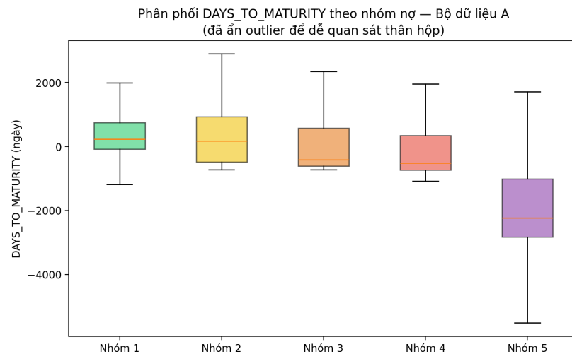
Hình 2.4: Phân phối DAYS_TO_MATURITY theo nhóm nợ — bộ dữ liệu A
