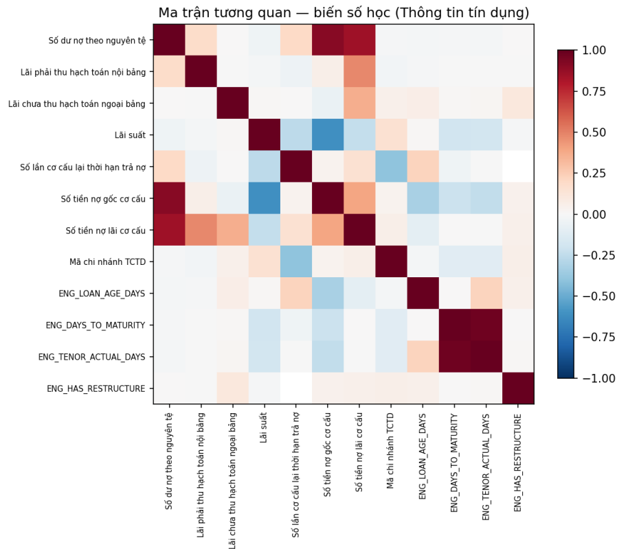
Hình 2.6: Ma trận tương quan giữa 12 biến số (8 biến gốc + 4 biến kỹ thuật) — bộ dữ liệu B
