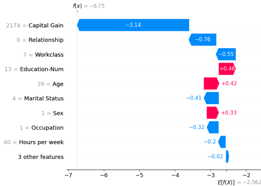
Hình 1.4: Ví dụ biểu đồ waterfall minh họa nguyên lý phân rã dự báo theo giá trị SHAP
