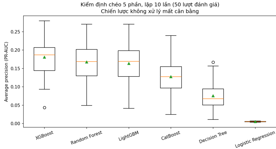
Hình 3.4: Phân tán PR-AUC qua 5 phần, lặp 10 lần kiểm định chéo — chiến lược none
