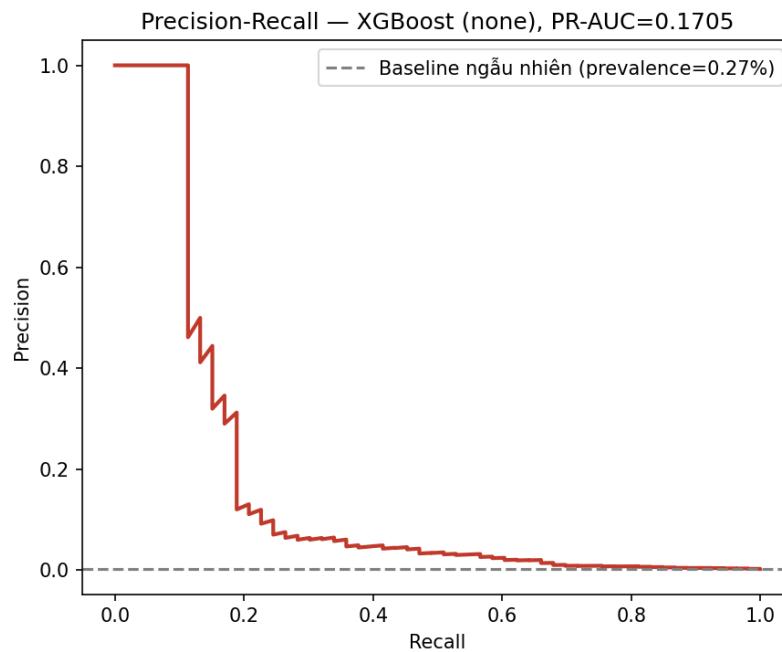
Hình 3.2: Đường cong Precision-Recall — XGBoost (none)
