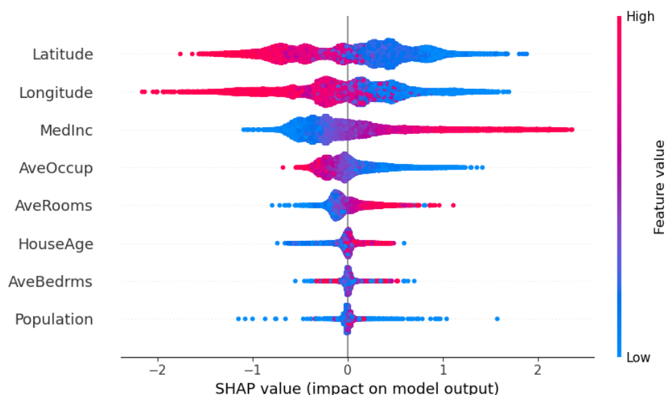
Hình 1.5: Ví dụ biểu đồ SHAP beeswarm trong phân tích mức độ tác động của đặc trưng
