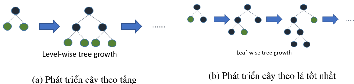
Hình 1.3: Minh họa hai chiến lược phát triển cây quyết định
