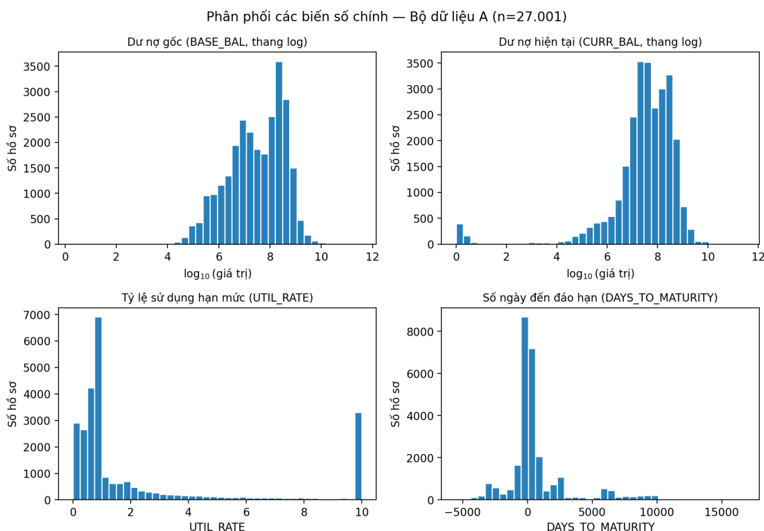
Hình 2.2: Phân phối bốn biến số chính của bộ dữ liệu A (n=27.001)
