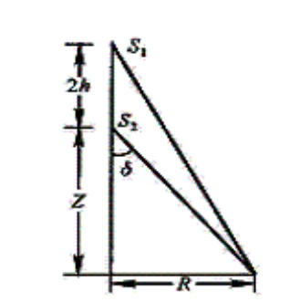
图 3 薄膜干涉计算示意图
