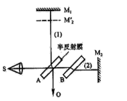
图 1 迈克尔逊干涉仪的原理图
