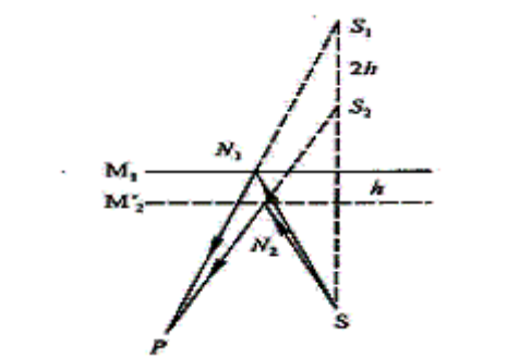
图 2 点光源的薄膜干涉
