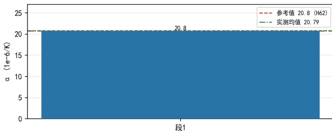
图 6 各段线膨胀系数与参考值对比 (实测均值 20.79 \times 10^{-6}/K , 参考 20.8)
