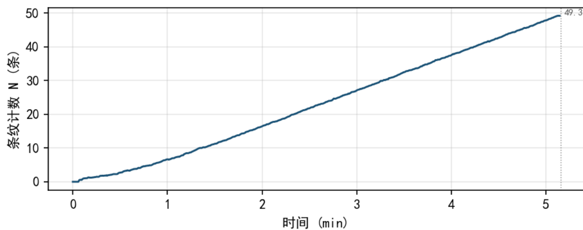
图 4 条纹计数曲线 N(t) (每段计数独立累计, 段末结算); 人工参考 52 条 vs 机器 49.27 条
