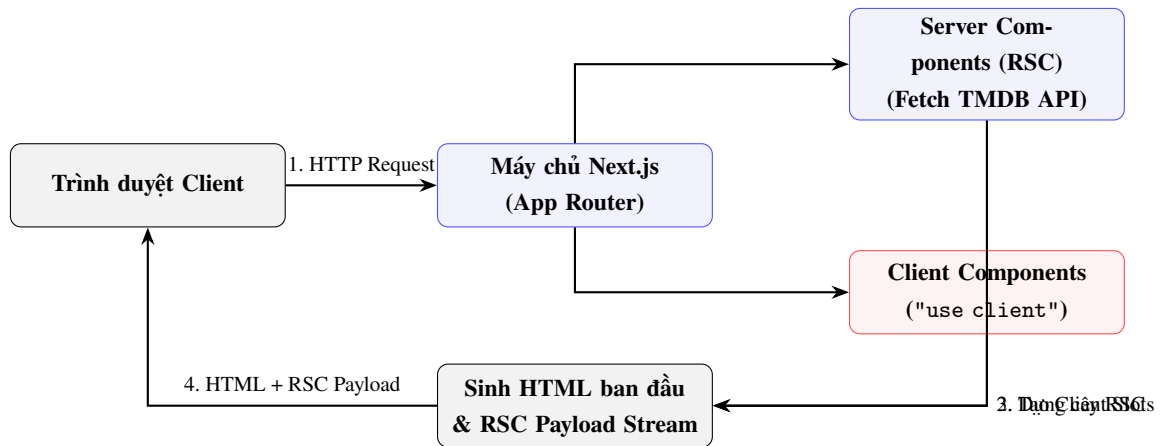
Hình 1.1. Sơ đồ luồng kết xuất React Server Components và đóng gói RSC Payload (Nguồn: Xây dựng dựa trên đặc tả kỹ thuật RSC [7])
