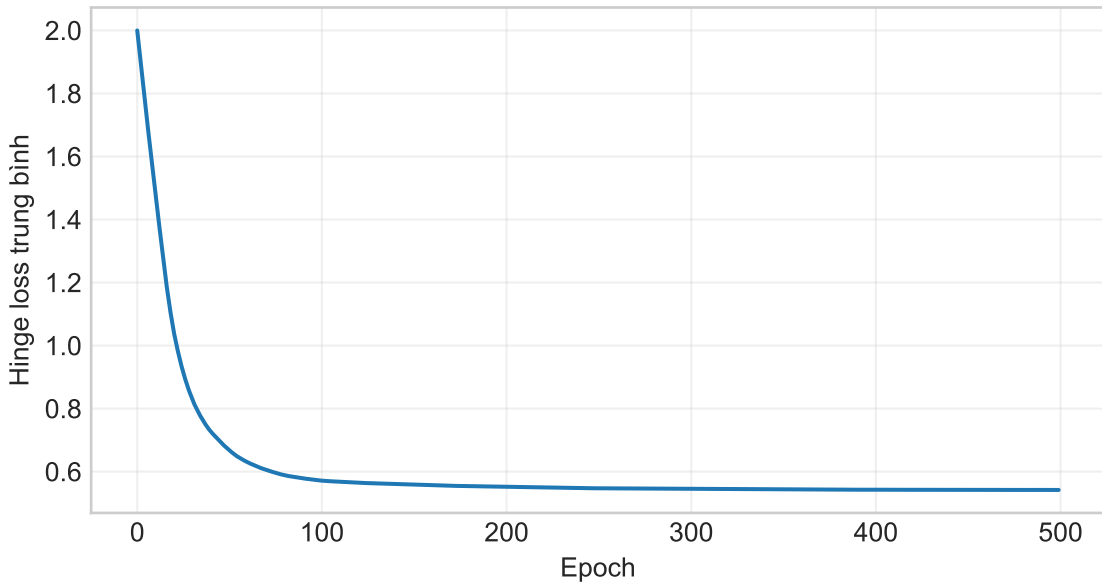
Hội tụ của Multi-class SVM (subgradient descent)
