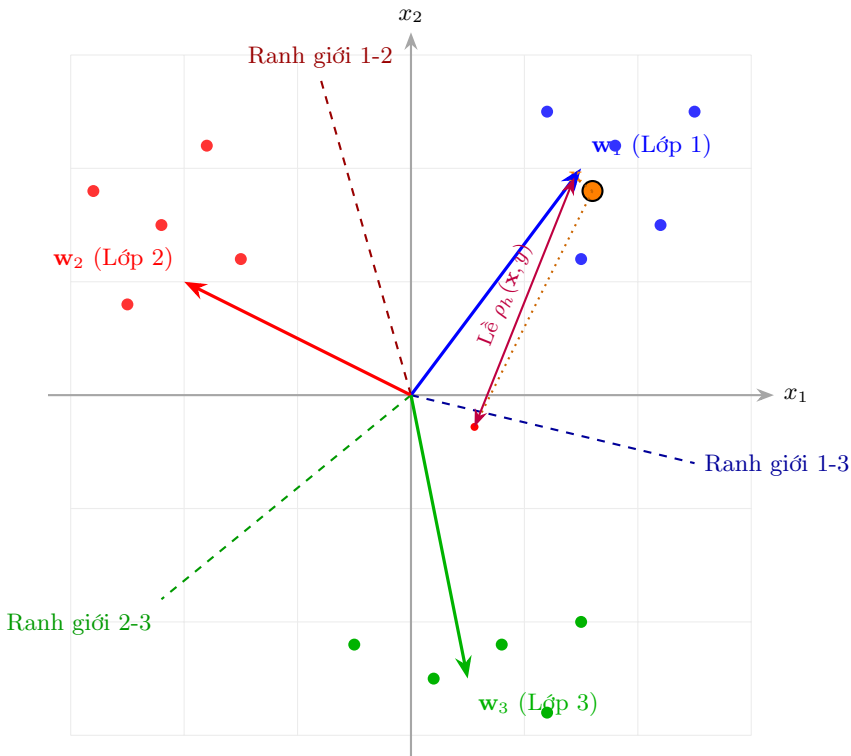
Hình 1.3.1: Ranh giới quyết định & Lệ của Multi-class SVM \mathbf{x} được gán nhãn \hat{y} = \arg \max_y (\mathbf{w}_y \cdot \mathbf{x}) (Hình chiếu lớn nhất)
