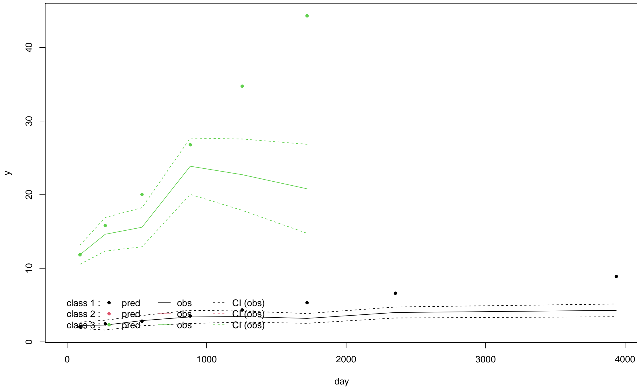
Class-specific bilirubin trajectories (K=3)
