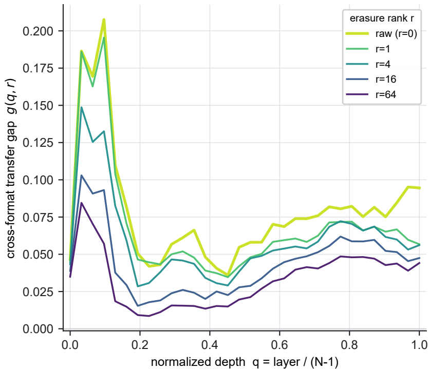
Llama-3.1-8B (N=32 layers)
