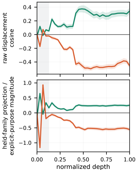
Llama 3.1 8B
