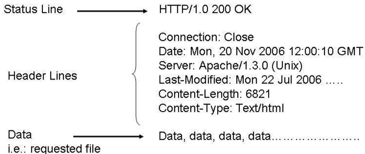
Fig. 8.3: Esempio di messaggio di risposta HTTP
