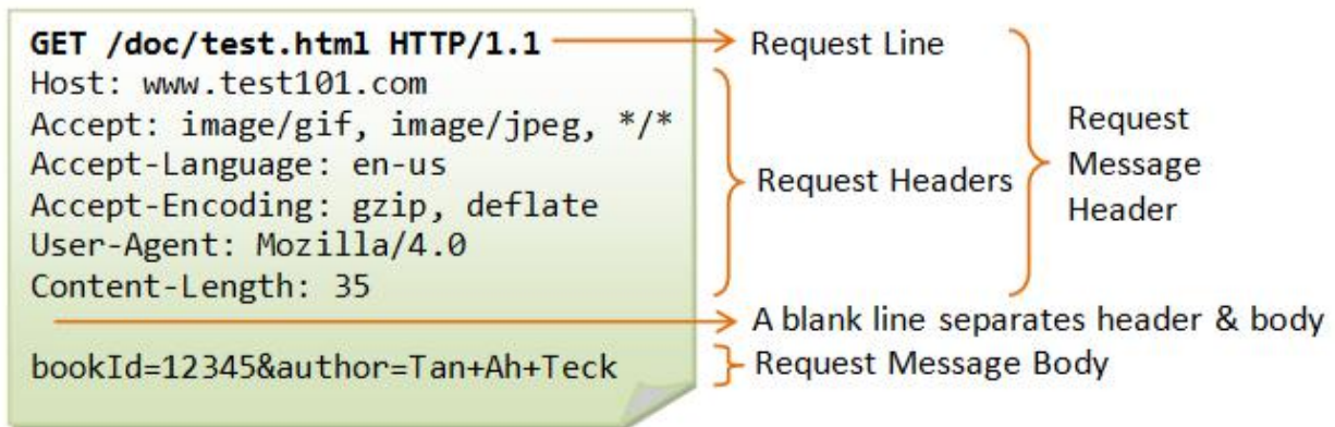
Fig. 8.2: Esempio di richiesta HTTP
