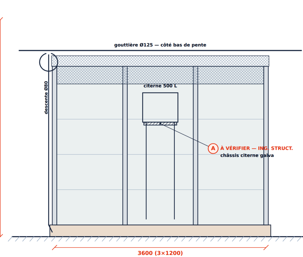
3 · ÉLÉVATION MUR LONG ARRIÈRE (côté bas) éch. ≈ 1:24
