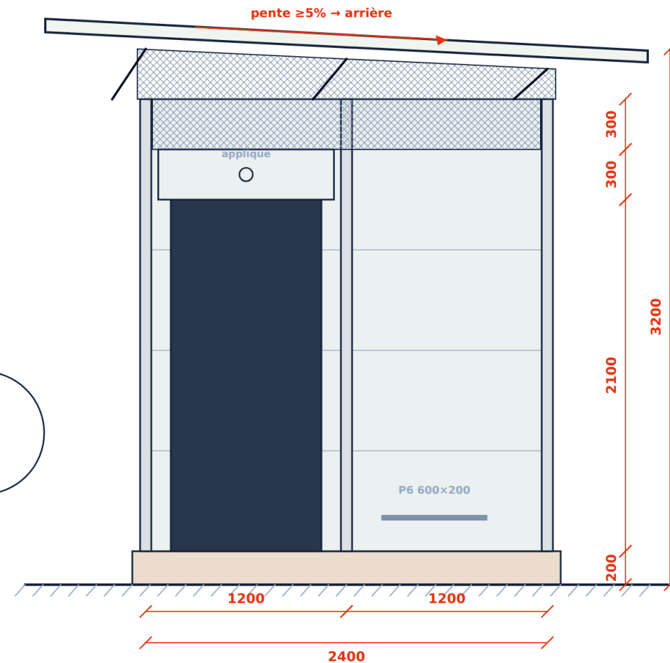
2 · ÉLÉVATION PIGNON (entrée H) éch. ≈ 1:20
