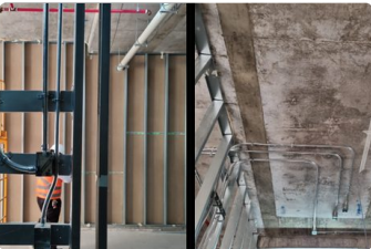
Nivel -1 Foto 11. Avance de canalizaciones eléctricas, 25-09-2026
