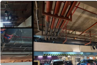
Conexión con edificio existente Foto 14. Avance de red hidrónica AC/AF, 28-09-2026
