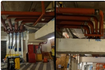
Conexión con edificio existente Foto 15. Avance de red hidrónica AC/AF, 28-09-2026
