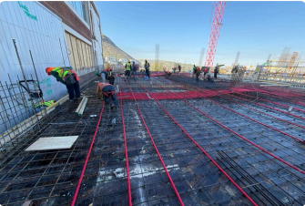
Losa cielo nivel 3 oriente
