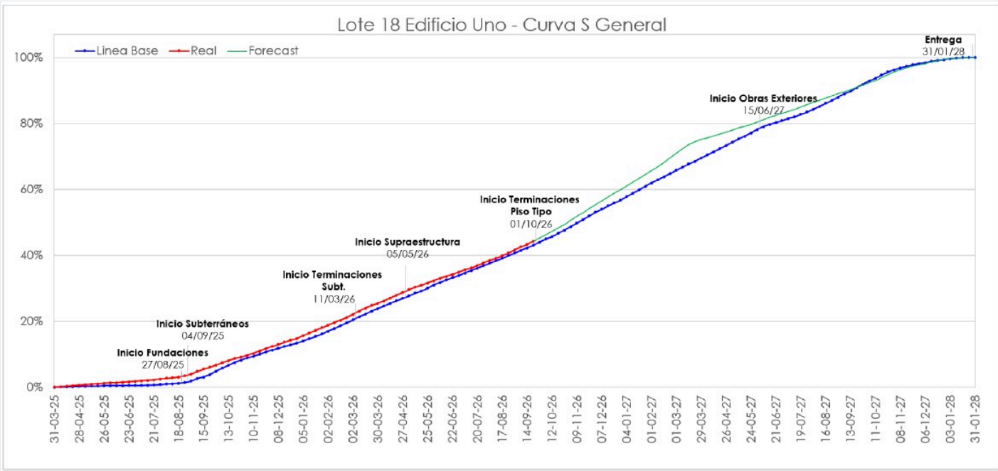
Curva S general del proyecto, con línea base, avance real y proyección hasta la entrega.
