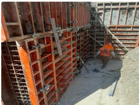
Piso -9 Moldaje de muros
