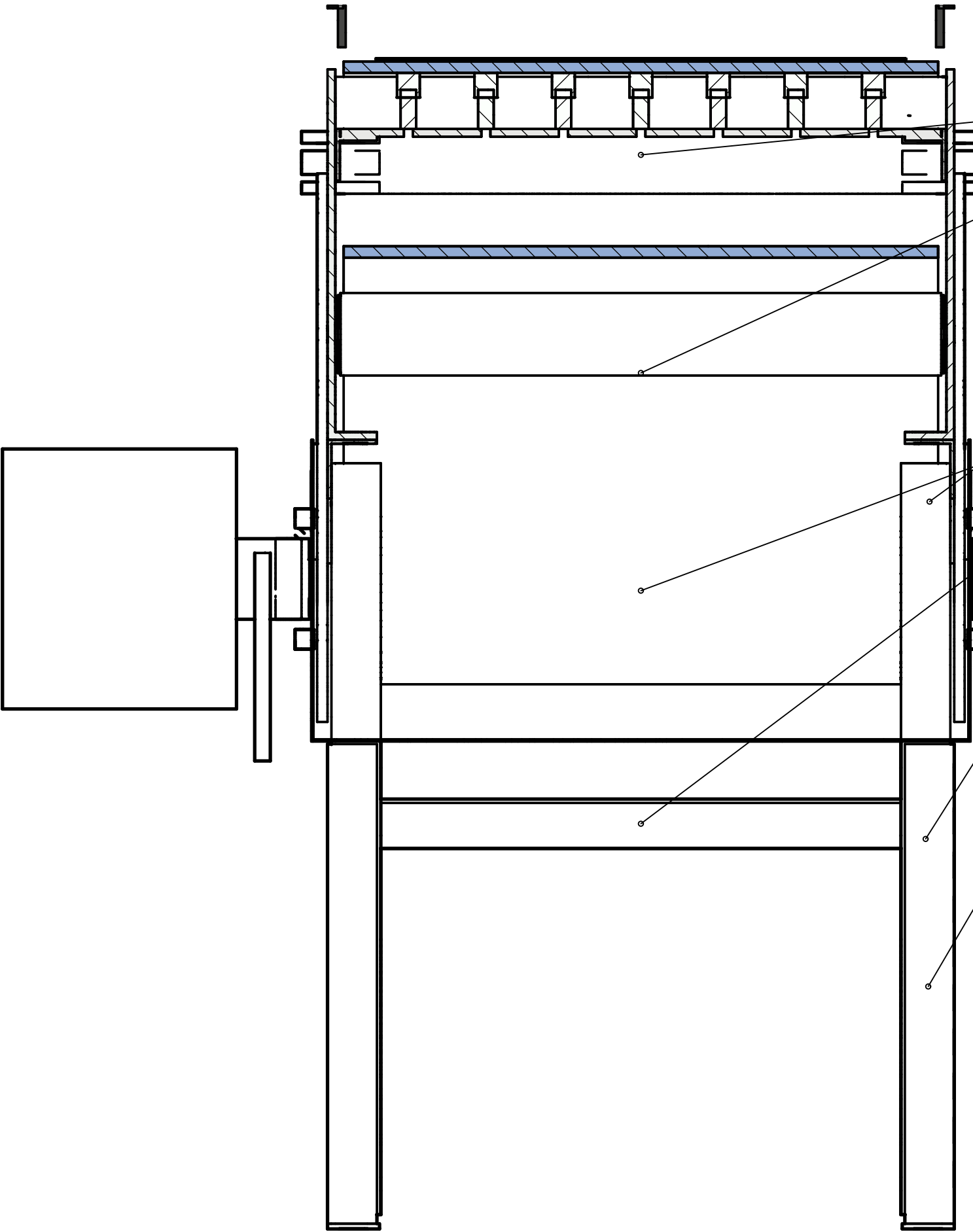
SECCIÓN A-A — transversal por portacarril (x=301) · ESC 1:3.8
