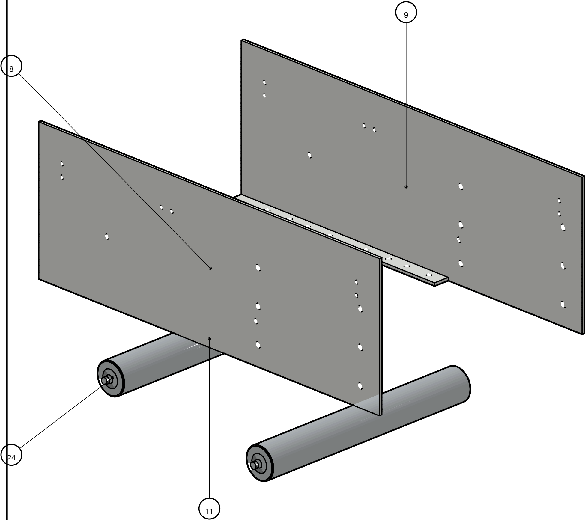
FIGURA B — RETORNO — RODILLOS DE EJE MUERTO
