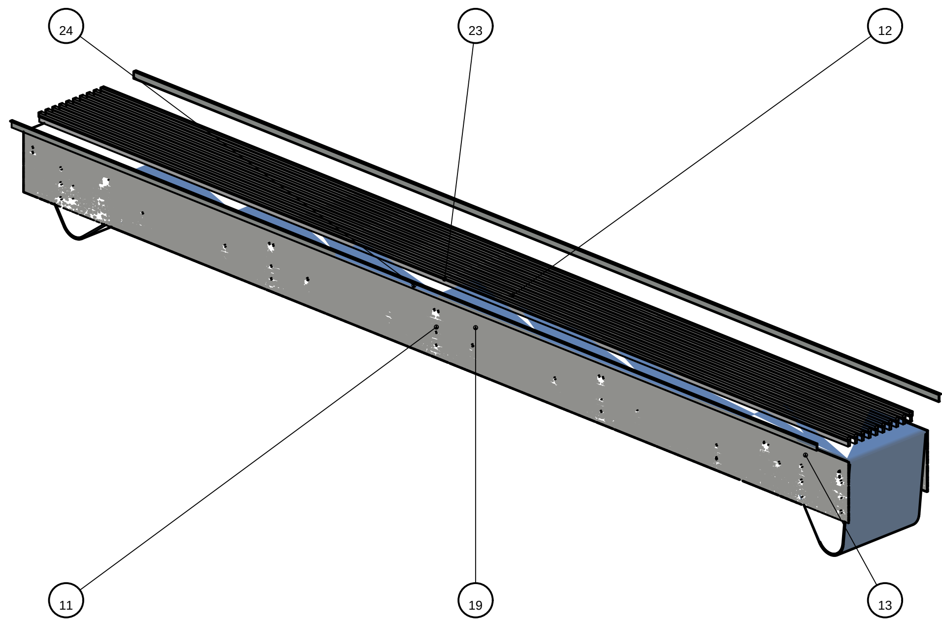
FIGURA G — CARRYWAY — BANDA Y GUÍAS
