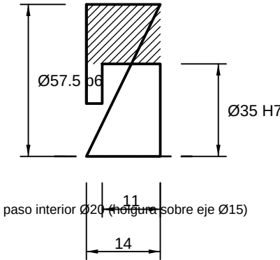
DETALLE CABEZAL (1:1) — media sección
