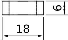
ALZADO
