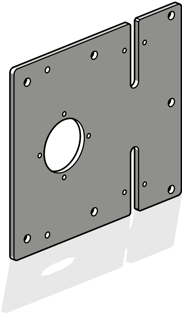
ISOMÉTRICA (pintada — referencia)
