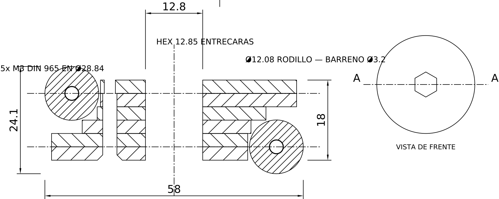
CORTE A-A (escala 2:1)
