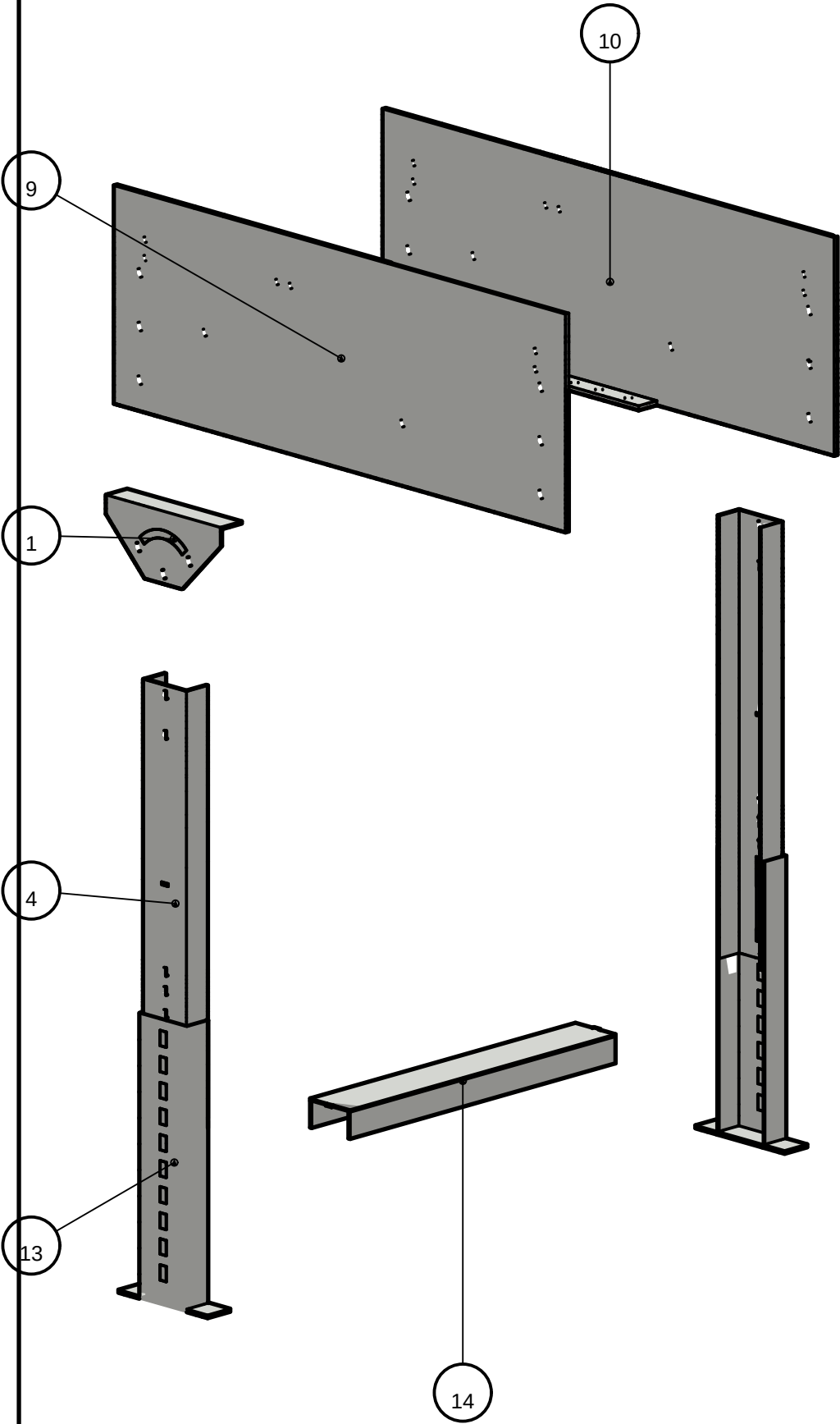
FIGURA H — SOPORTES A PISO — SISTEMA 24V
