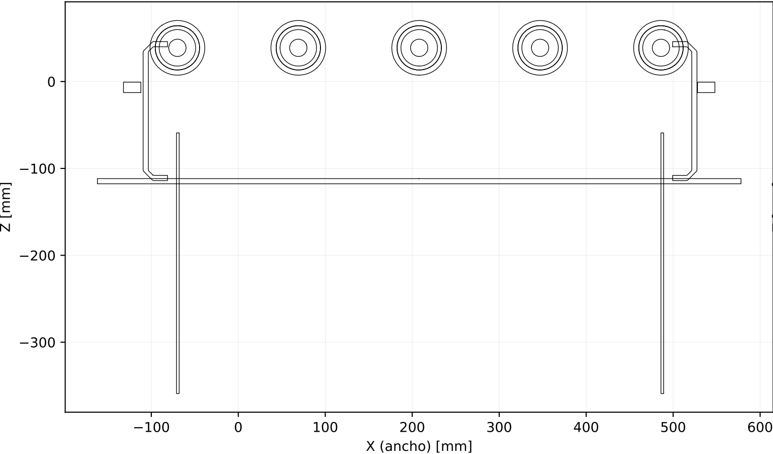
Corte transversal B-B (plano Y=-1090, por la transferencia)
