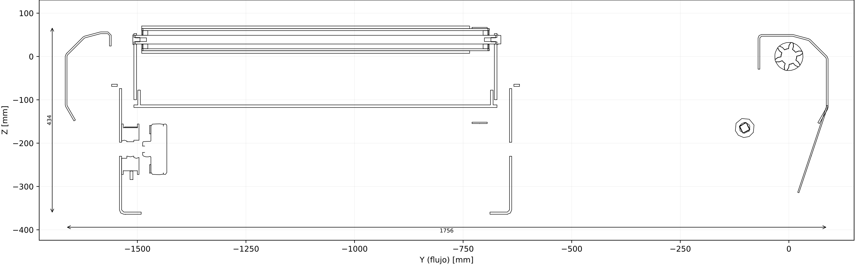
Corte longitudinal A-A (plano X=208, eje de máquina)
