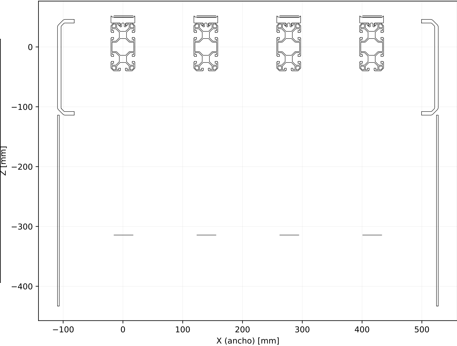
Corte transversal C-C (plano Y=-300, por cabezal motriz)
