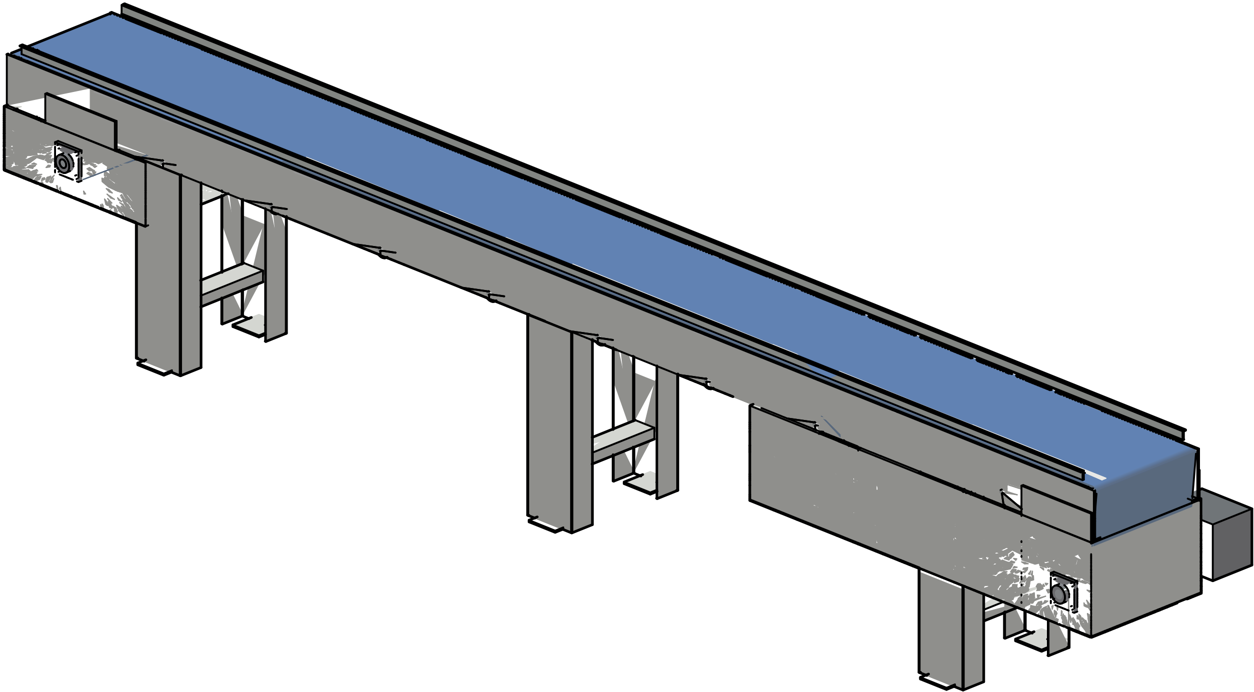
Largo nose a nose: 5000 mm · Ancho total ~498 mm · Faja superior a nivel de placas Banda y rodillos LBP no ilustrados en detalle (ver Figura G). Escala gráfica — no medir sobre la figura.
