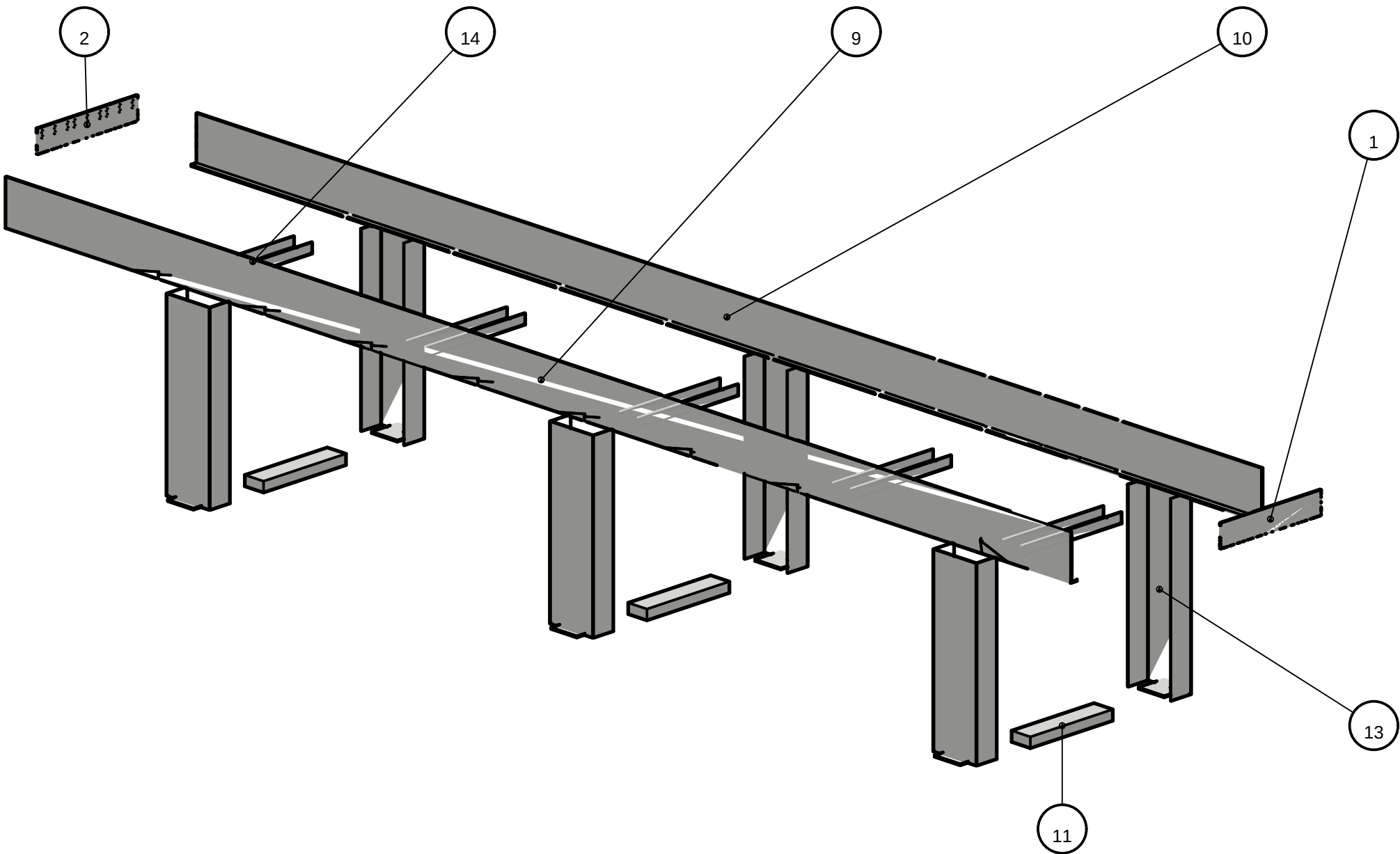
FIGURA A — BASTIDOR SOLDADO Y ESTRUCTURA
