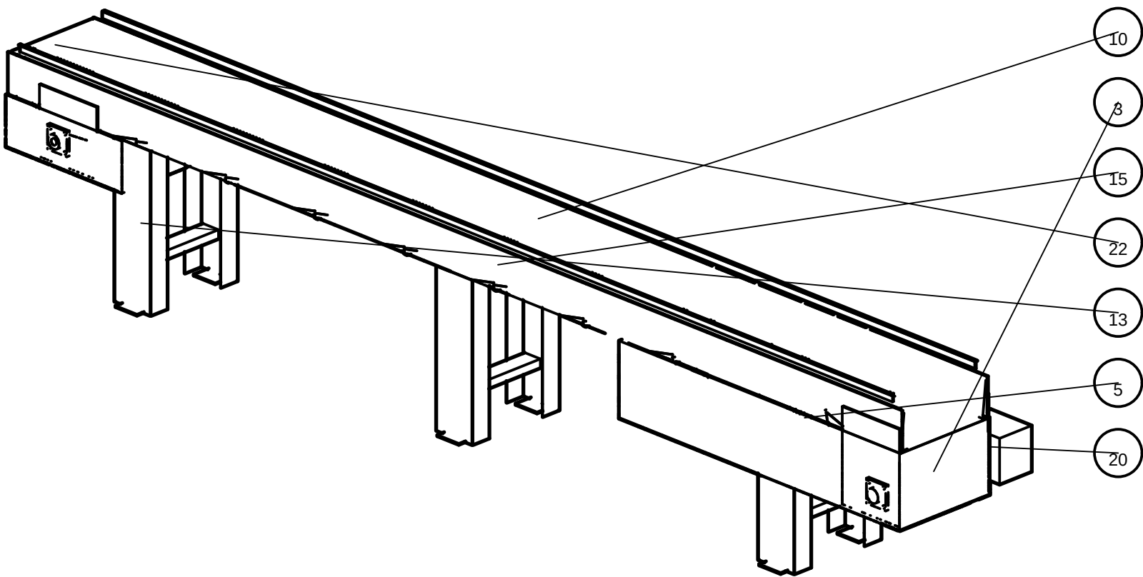
ISOMÉTRICA (referencia)
