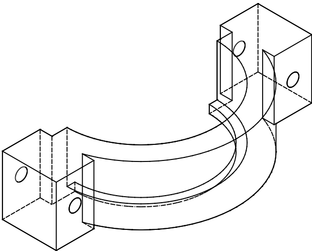
ISOMÉTRICA
