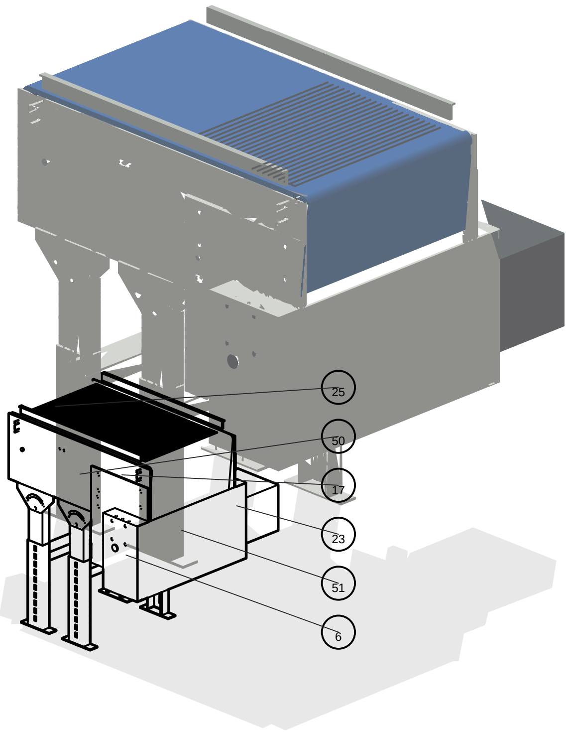
ISOMÉTRICA (referencia)
