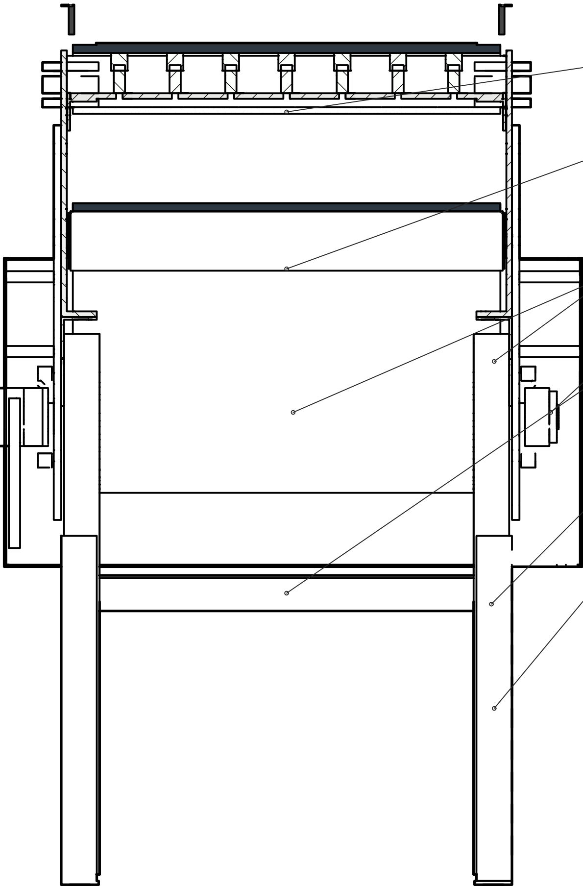
SECCIÓN A-A — transversal por portacarril (x=301) · ESC 1:4.0
