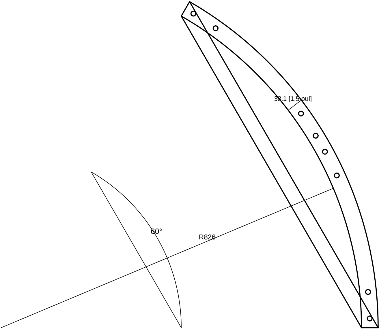
CORTE PLANO (sector de corona — no se desarrolla)
