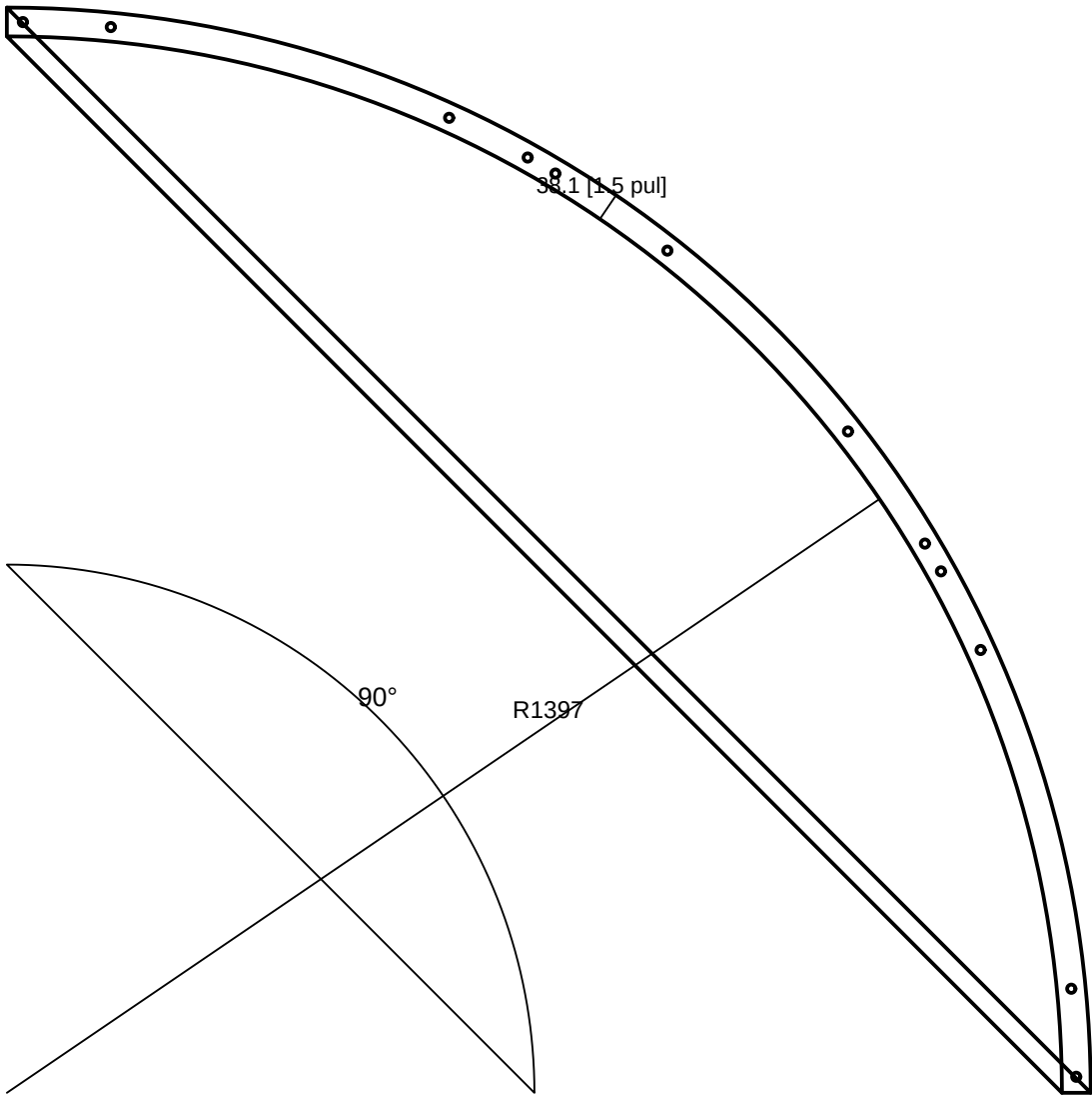
12 barrenos · Ø 11 CORTE PLANO (sector de corona — no se desarrolla)
