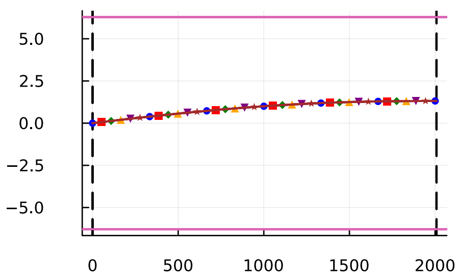
\phi
