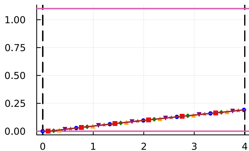
x_3
