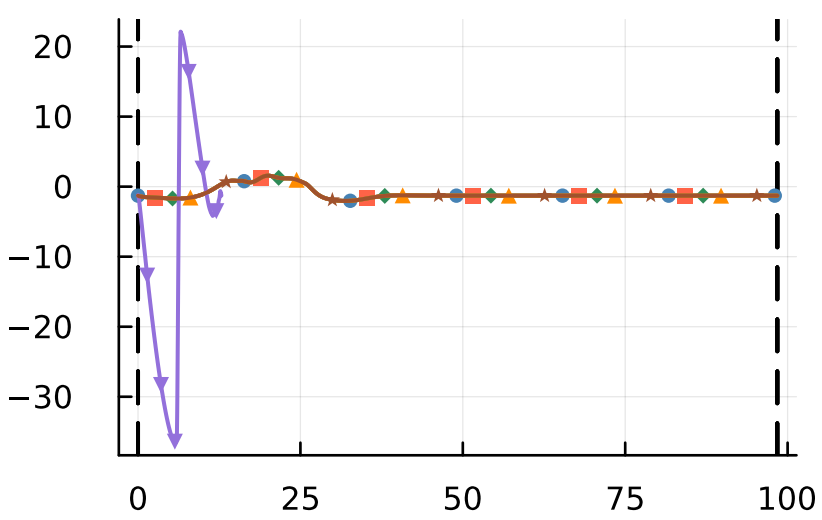
vy
