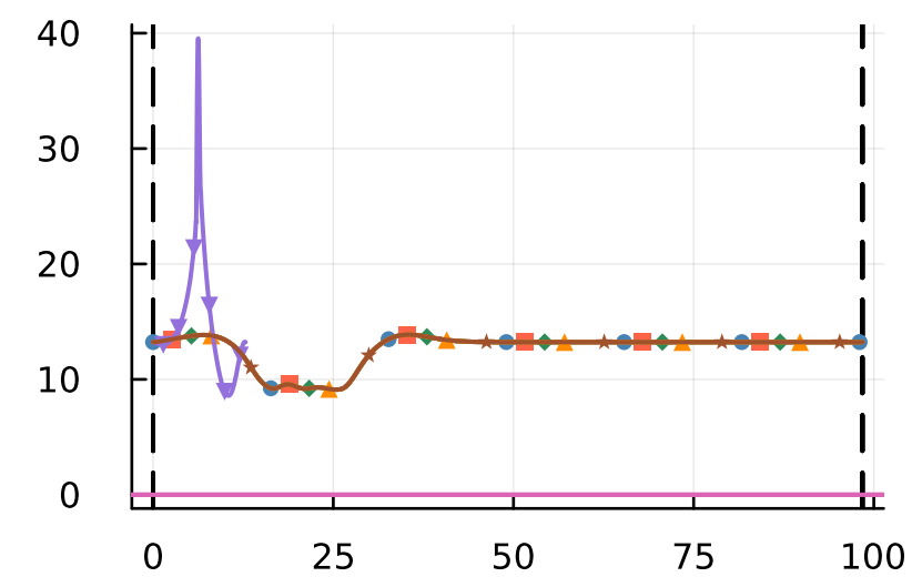
vx
