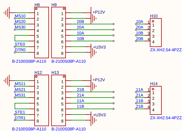
执行器02：步进电机
