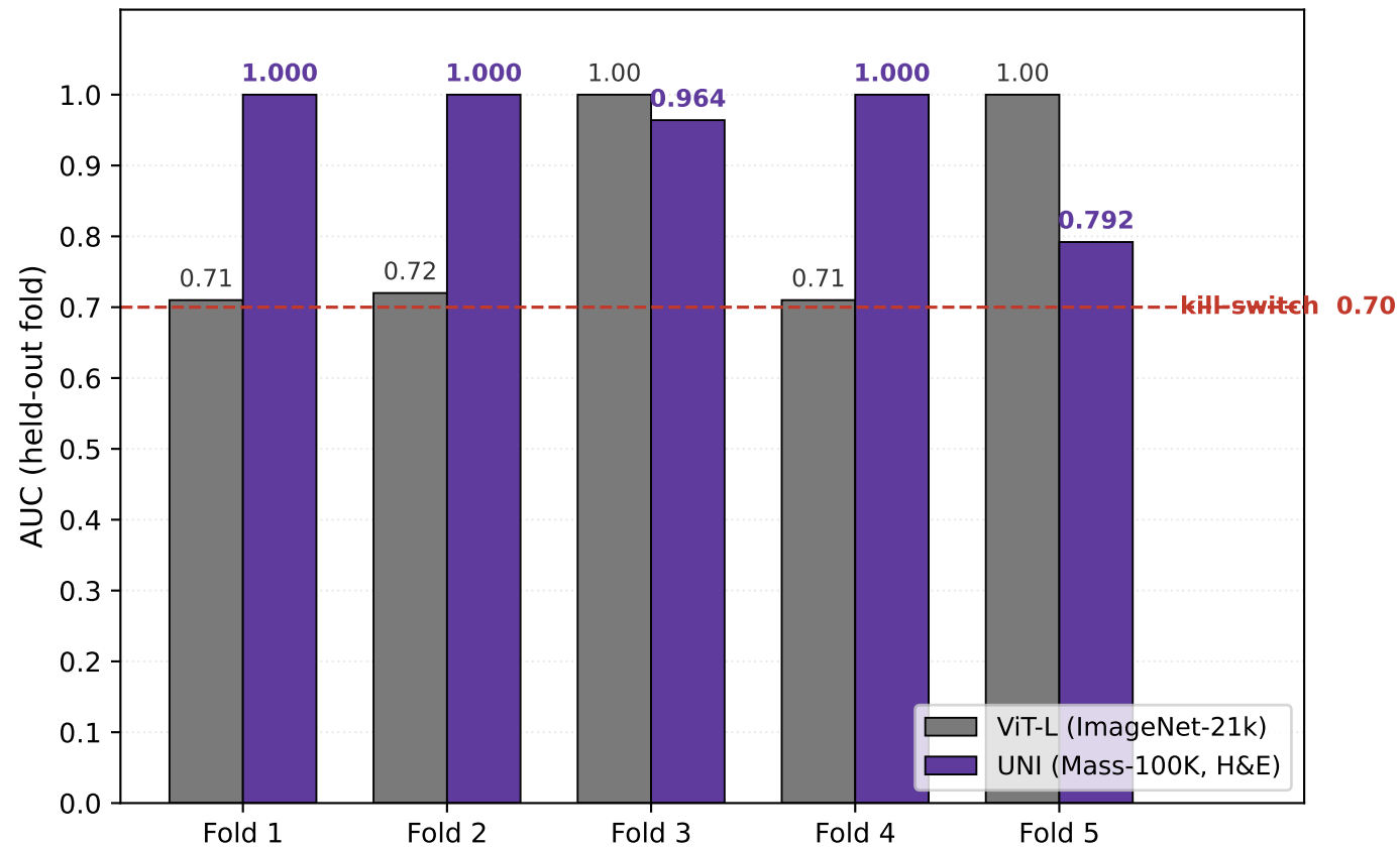
A. Per-fold AUC — ViT-L vs UNI
