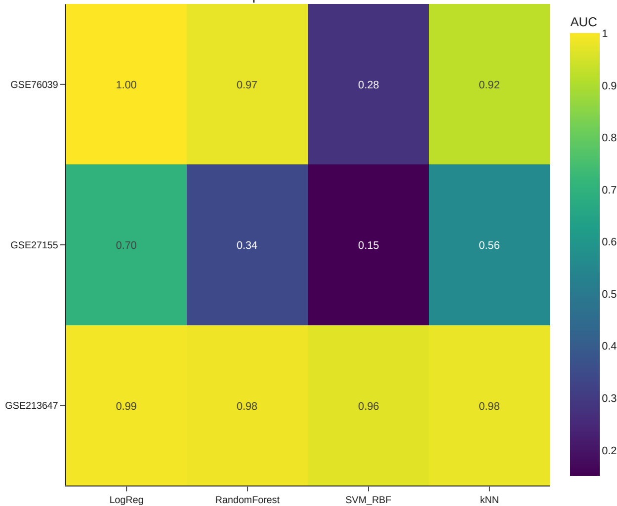
AUC per cohort × classifier
