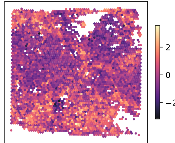
GSM7980869_LPTC-2 ITD-1
