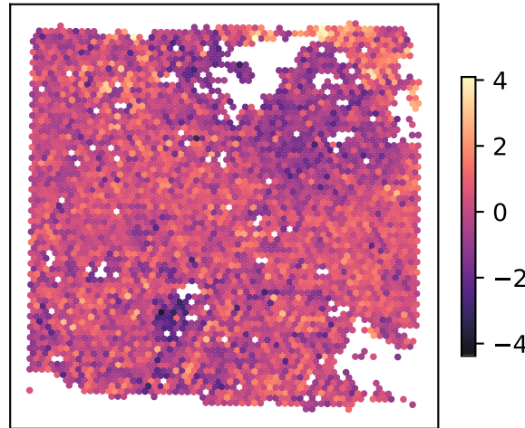
GSM7980869_LPTC-2 AZ 628
