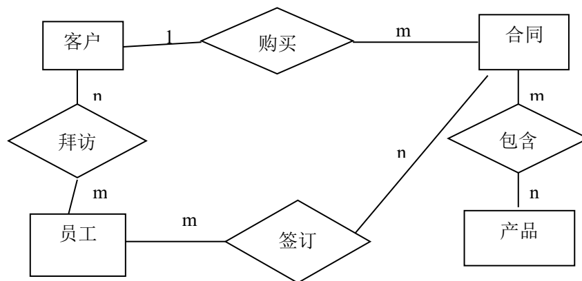
图 3.1 销售业务管理系统 E-R 图
